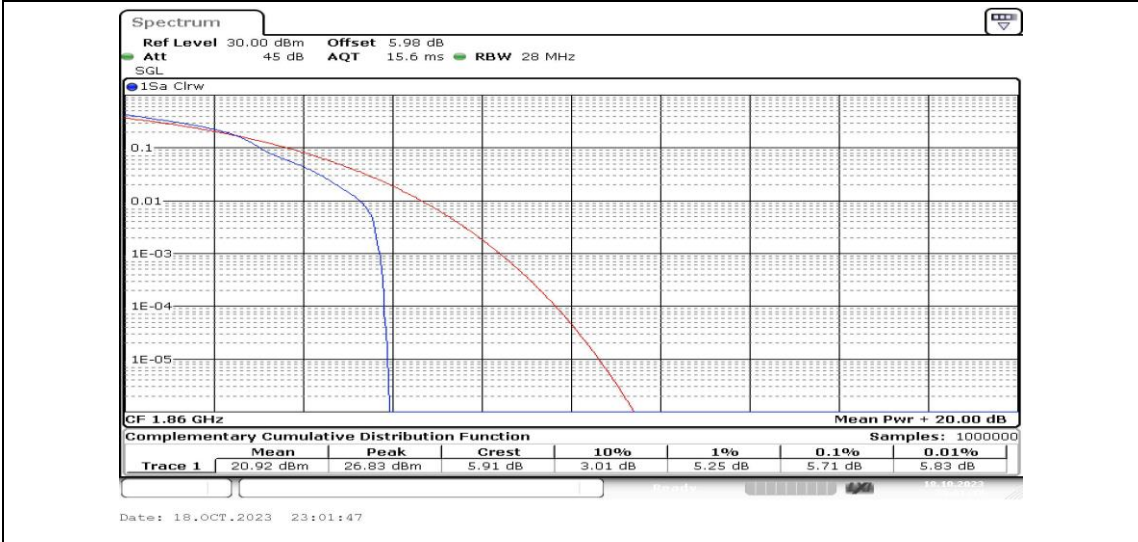
Band2-20MHz-16QAM-18700-1RB#0-PASS
