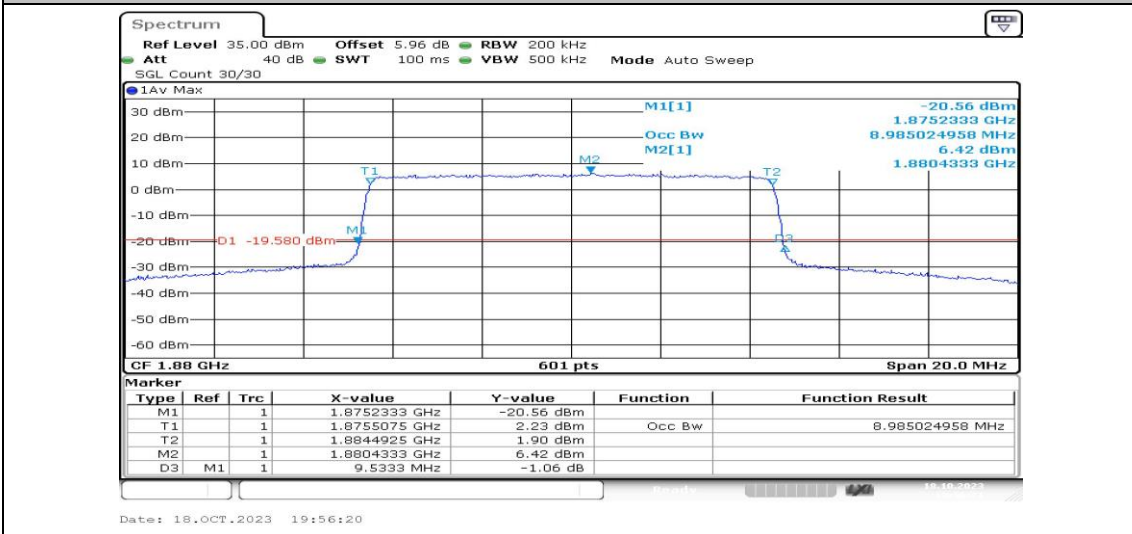
Band2-10MHz-QPSK-18900-50RB#0-PASS
