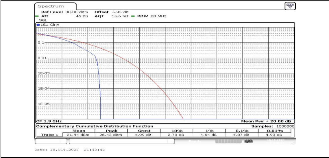
Band2-20MHz-QPSK-19100-1RB#0-PASS
