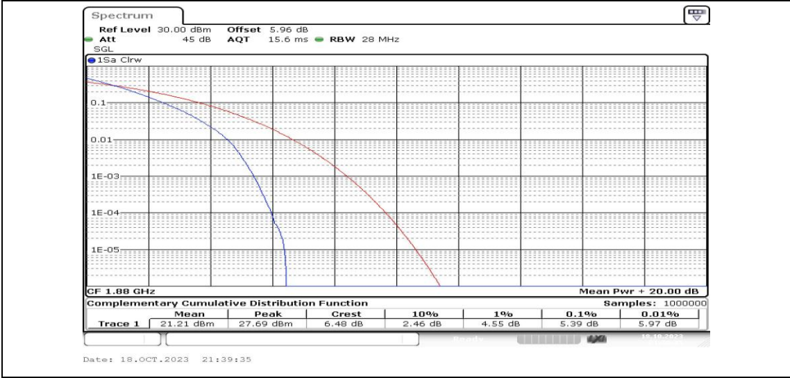
Band2-20MHz-QPSK-18900-100RB#0-PASS
