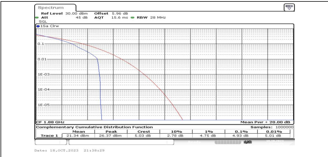
Band2-20MHz-QPSK-18900-1RB#0-PASS
