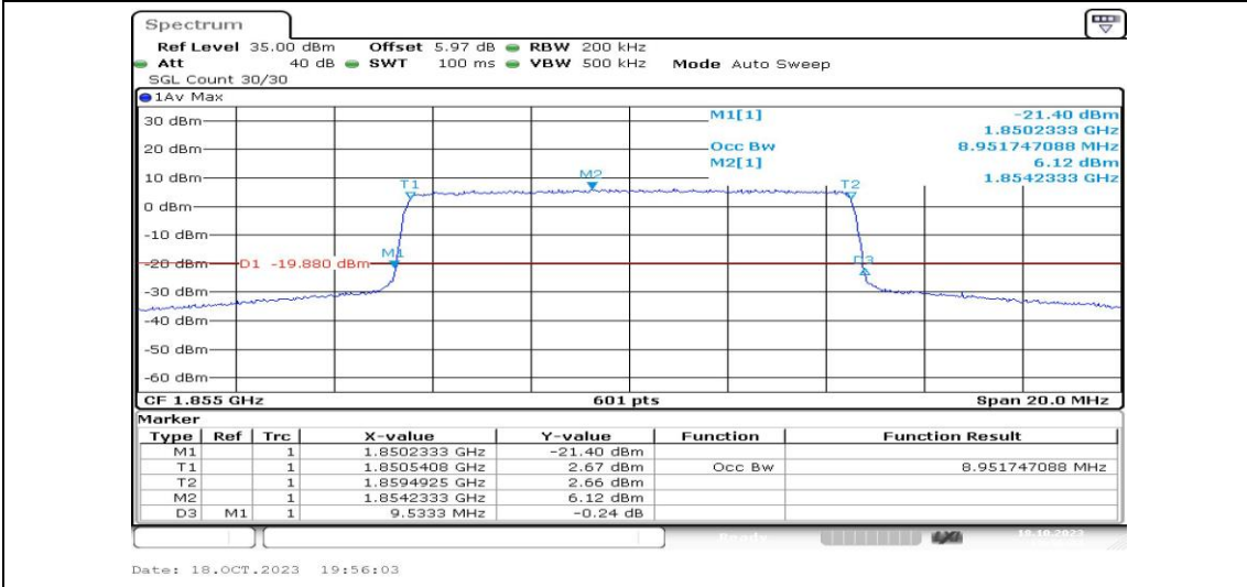
Band2-10MHz-QPSK-18650-50RB#0-PASS
