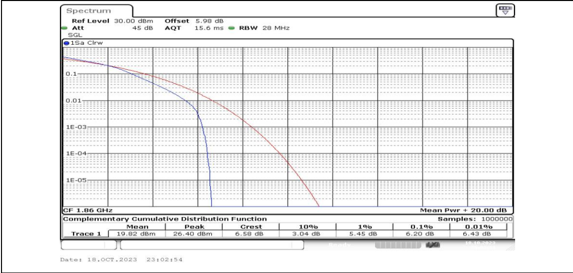
Band2-20MHz-16QAM-18700-25RB#0-PASS
