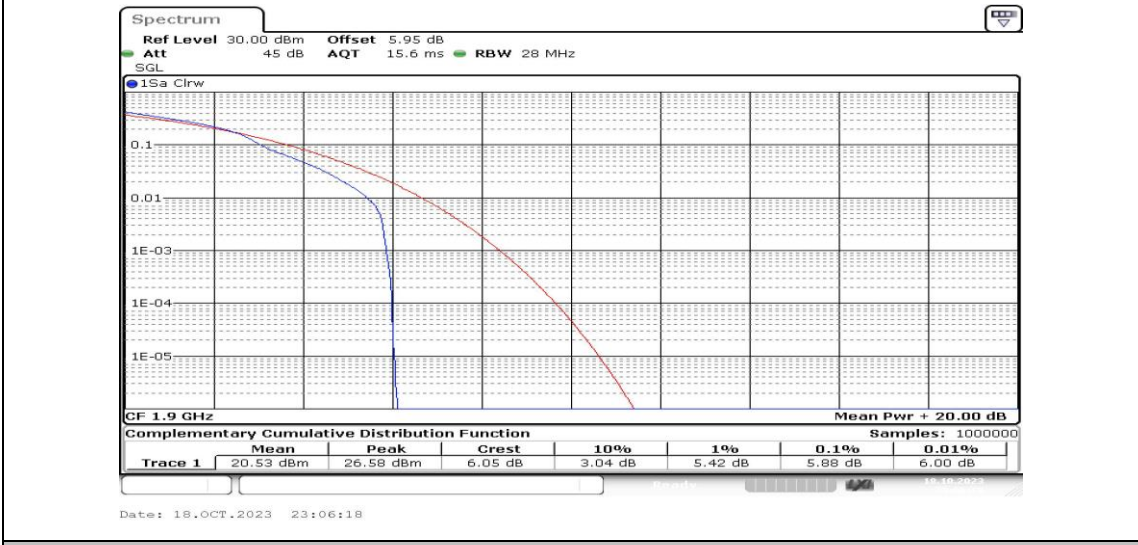
Band2-20MHz-16QAM-19100-1RB#0-PASS
