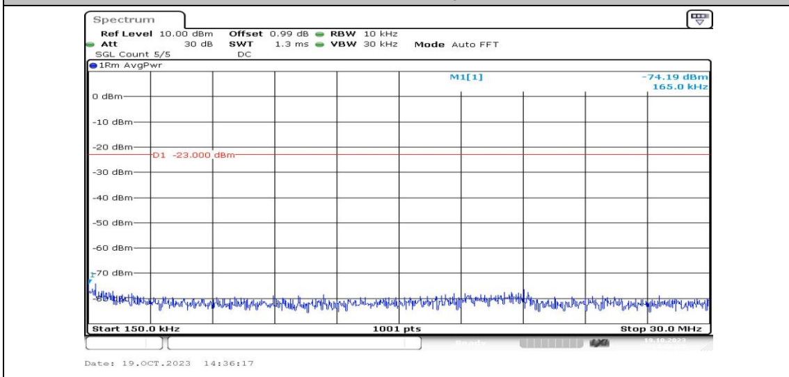
Band26-5MHz-QPSK-26715-1RB#0-Range2:0.15~30MHz-PASS
