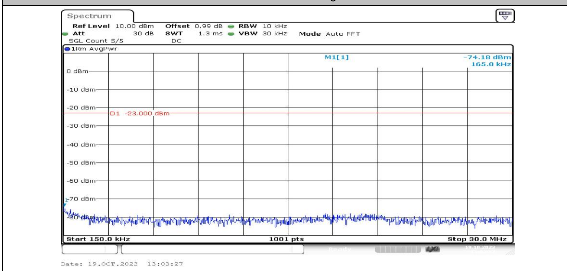
Band26-1.4MHz-QPSK-26697-1RB#0-Range2:0.15~30MHz-PASS
