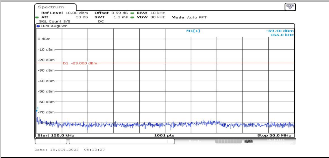
Band25-20MHz-QPSK-26140-1RB#0-Range2:0.15~30MHz-PASS
