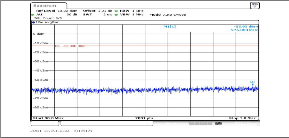
Band25-10MHz-QPSK-26365-1RB#0-Range3:30~1000MHz-PASS
