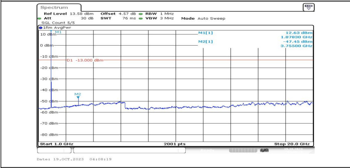
Band25-10MHz-QPSK-26365-1RB#0-Range4:1000~20000MHz-PASS
