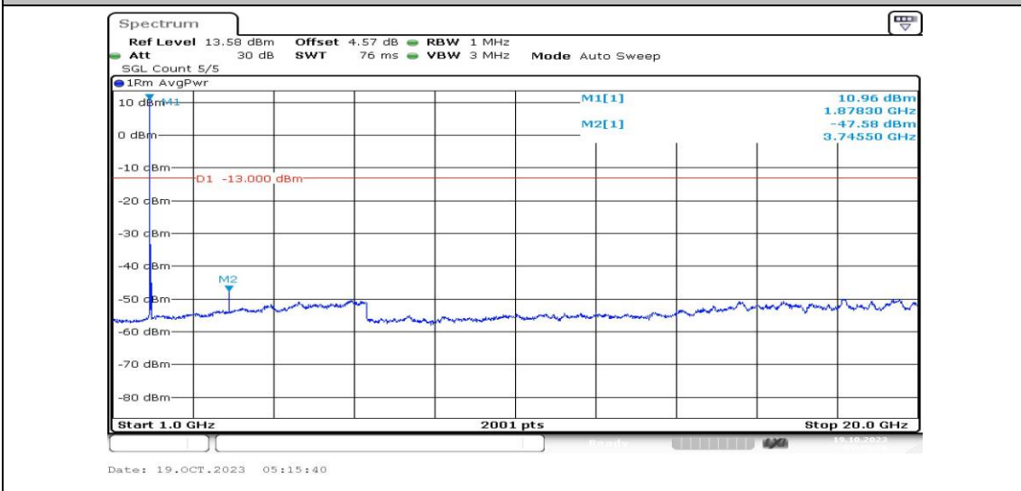
Band25-20MHz-QPSK-26365-1RB#0-Range4:1000~20000MHz-PASS
