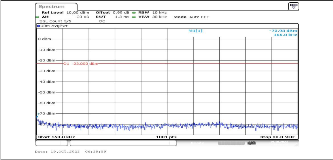
Band25-20MHz-16QAM-26590-1RB#0-Range2:0.15~30MHz-PASS
