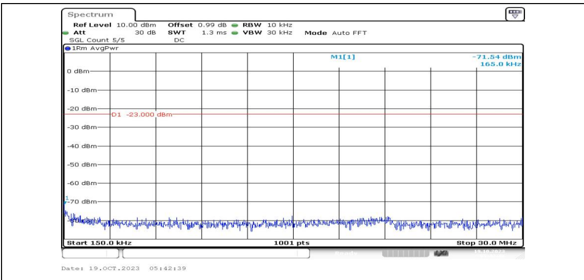
Band25-10MHz-16QAM-26365-1RB#0-Range2:0.15~30MHz-PASS
