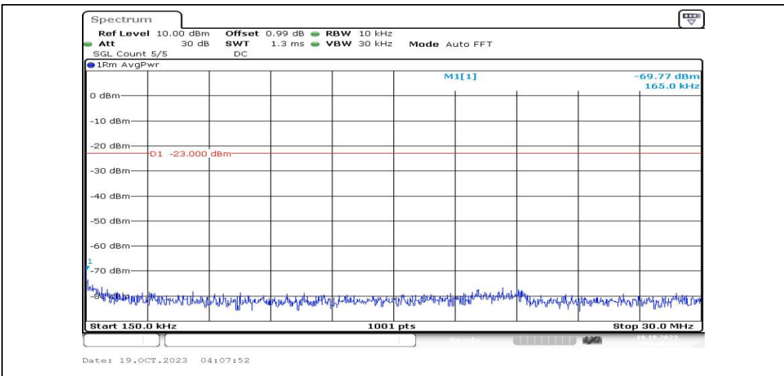
Band25-10MHz-QPSK-26365-1RB#0-Range2:0.15~30MHz-PASS
