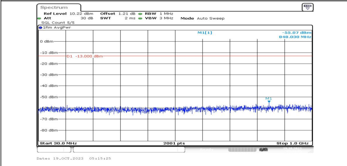
Band25-20MHz-QPSK-26365-1RB#0-Range3:30~1000MHz-PASS
