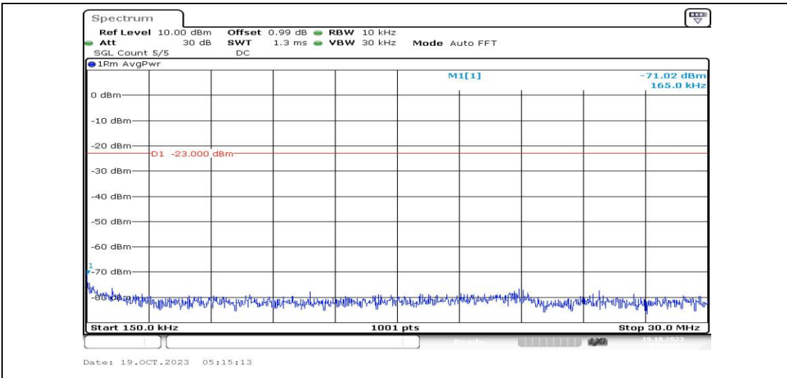
Band25-20MHz-QPSK-26365-1RB#0-Range2:0.15~30MHz-PASS
