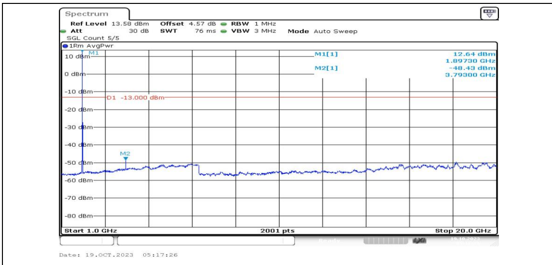
Band25-20MHz-QPSK-26590-1RB#0-Range4:1000~20000MHz-PASS
