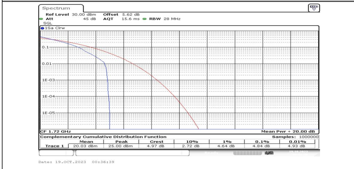
Band4-20MHz-QPSK-20050-1RB#0-PASS
