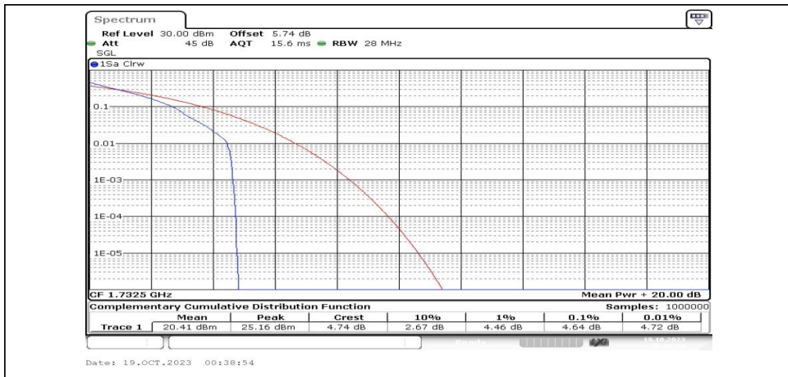
Band4-20MHz-QPSK-20175-1RB#0-PASS
