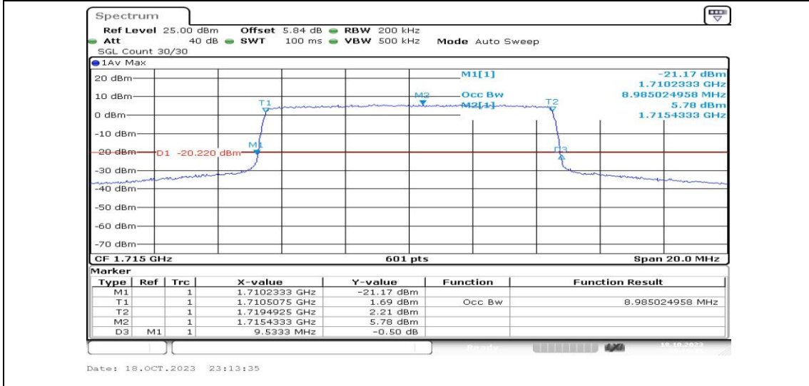
Band4-10MHz-QPSK-2000-50RB#0-PASS
