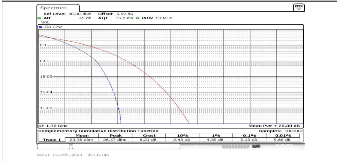
Band4-20MHz-QPSK-20050-100RB#0-PASS
