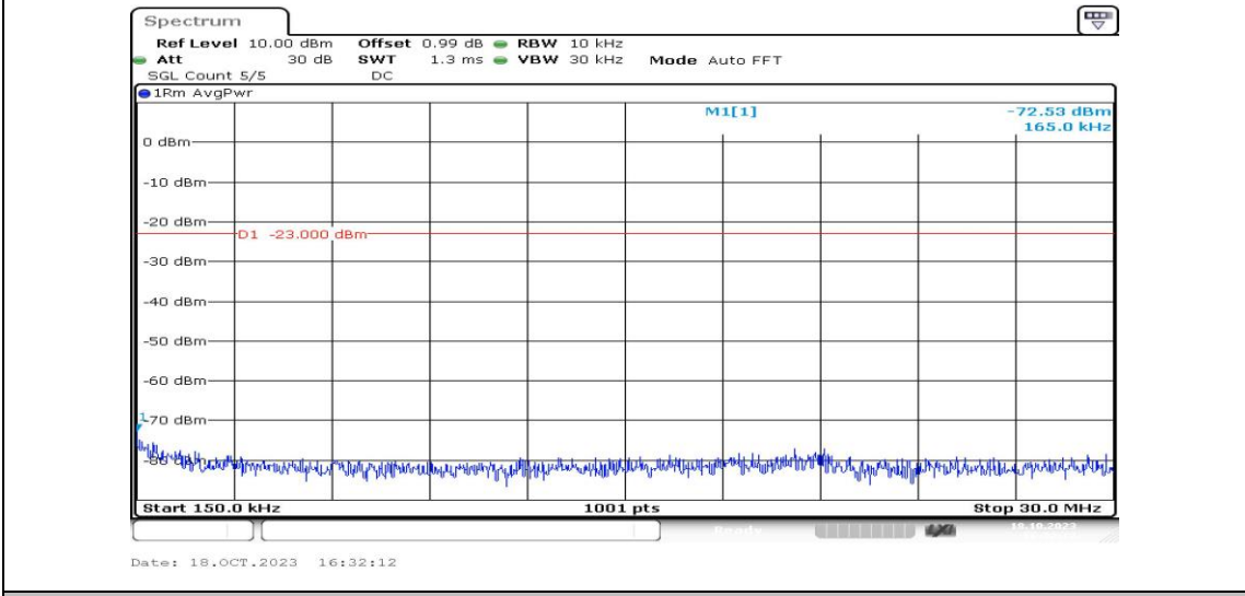
Band25-3MHz-16QAM-26365-1RB#0-Range2:0.15~30MHz-PASS
