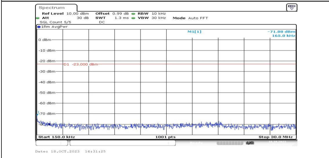
Band25-3MHz-QPSK-26365-1RB#0-Range2:0.15~30MHz-PASS
