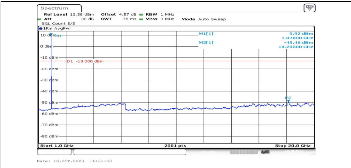
Band25-3MHz-QPSK-26365-1RB#0-Range4:1000~20000MHz-PASS
