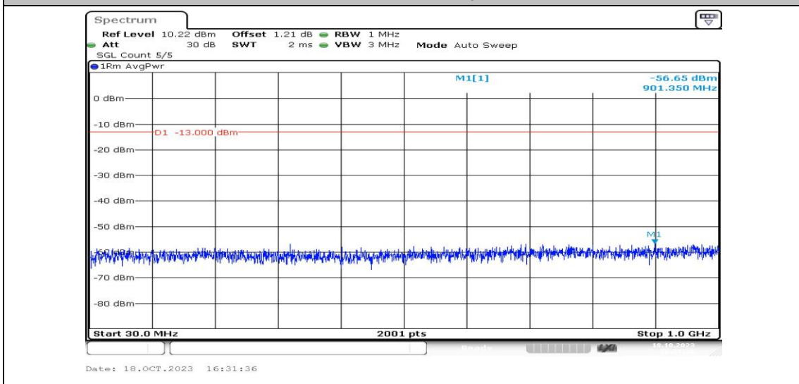
Band25-3MHz-QPSK-26365-1RB#0-Range3:30~1000MHz-PASS
