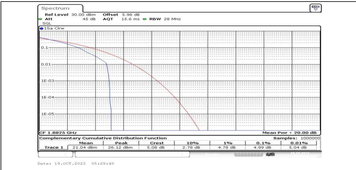
Band25-20MHz-QPSK-26365-1RB#0-PASS
