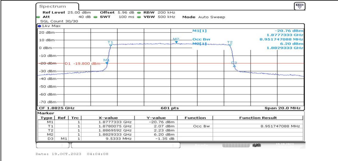
Band25-10MHz-QPSK-26365-50RB#0-PASS
