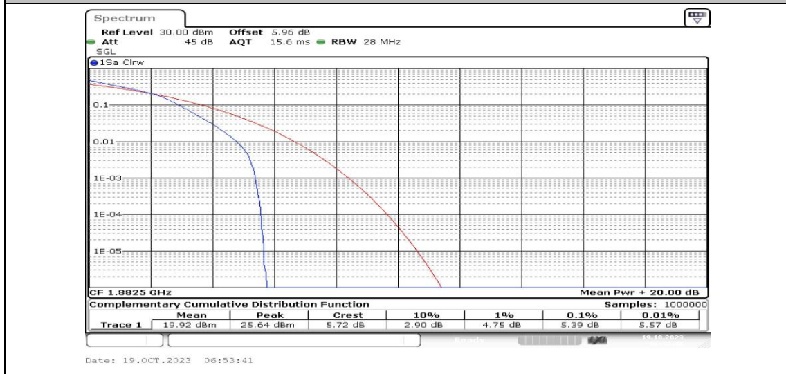
Band25-20MHz-16QAM-26365-25RB#0-PASS
