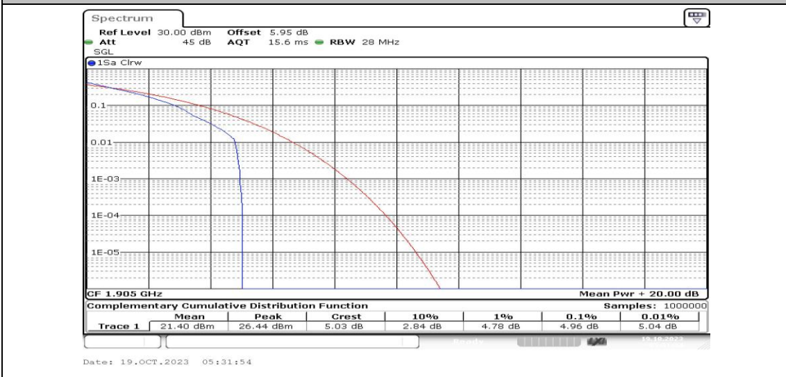
Band25-20MHz-QPSK-26590-1RB#0-PASS
