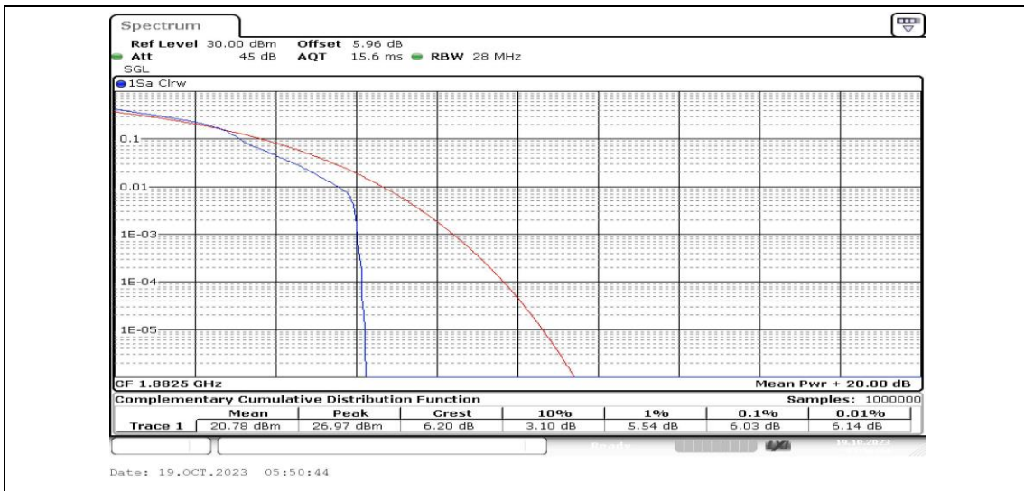
Band25-10MHz-16QAM-26365-1RB#0-PASS
