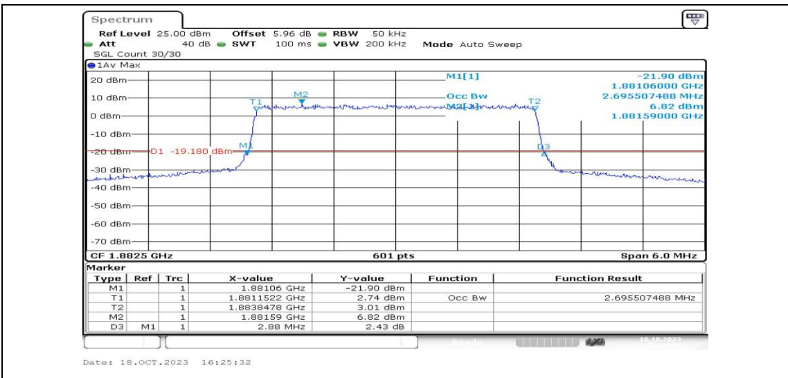
Band25-3MHz-QPSK-26365-15RB#0-PASS
