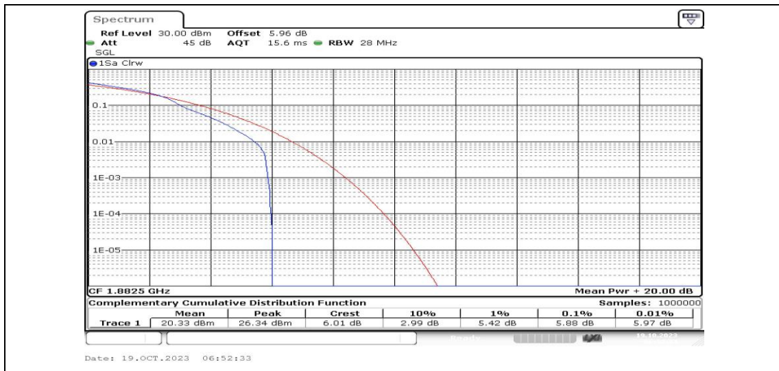
Band25-20MHz-16QAM-26365-1RB#0-PASS
