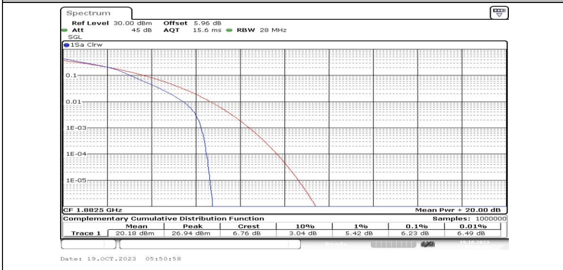
Band25-10MHz-16QAM-26365-25RB#0-PASS
