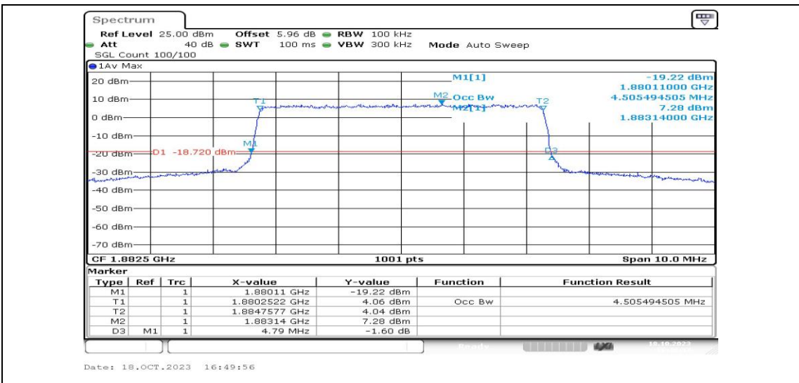
Band25-5MHz-QPSK-26365-25RB#0-PASS
