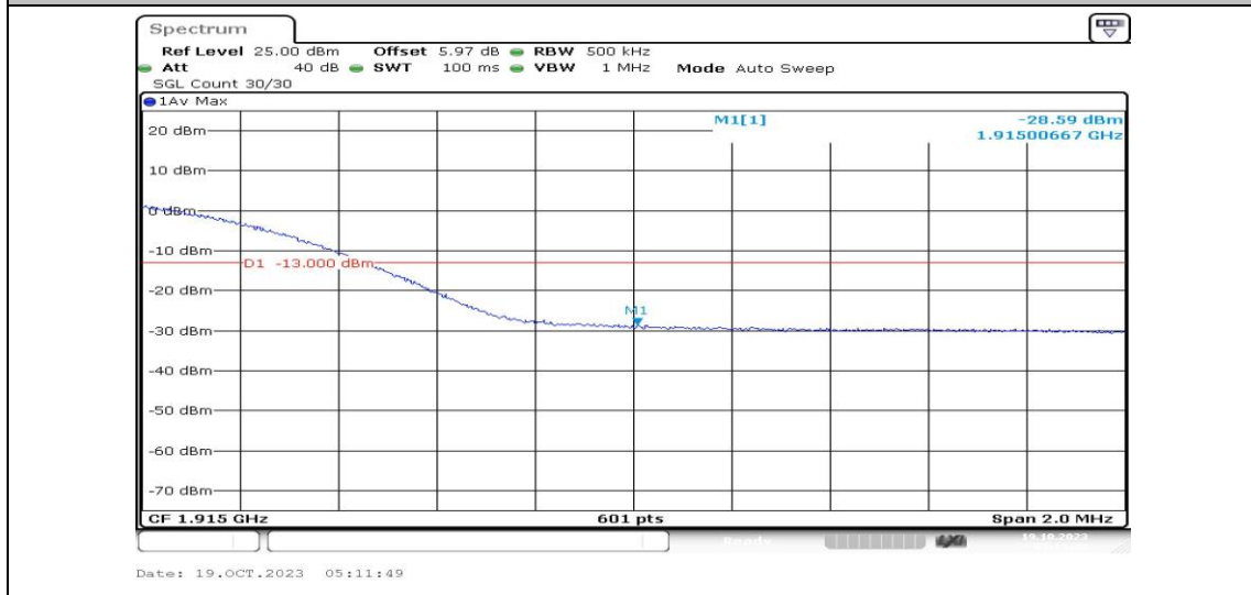
Band25-20MHz-QPSK-26590-100RB#0-PASS
