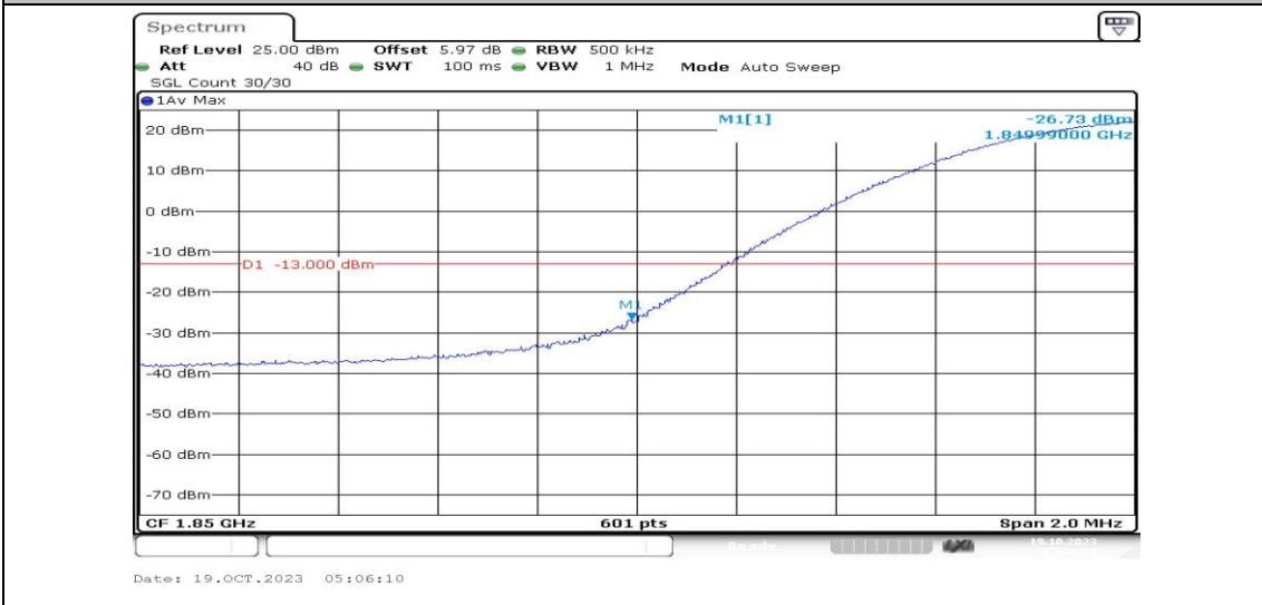
Band25-20MHz-QPSK-26140-1RB#0-PASS
