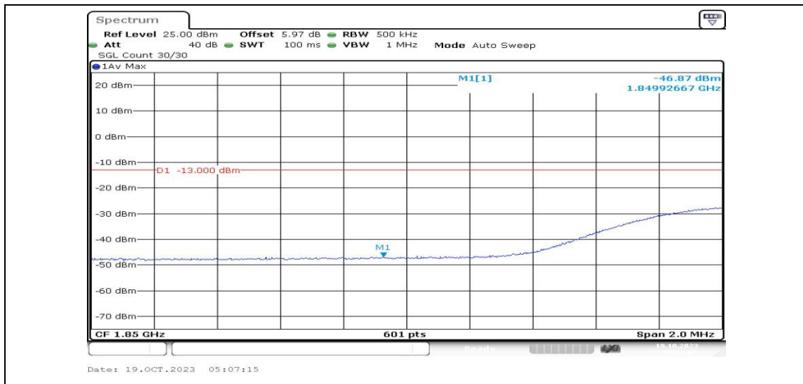
Band25-20MHz-QPSK-26140-1RB#99-PASS
