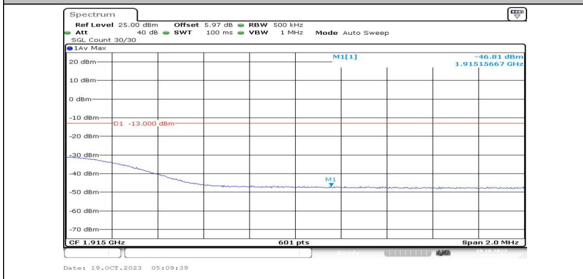
Band25-20MHz-QPSK-26590-1RB#0-PASS
