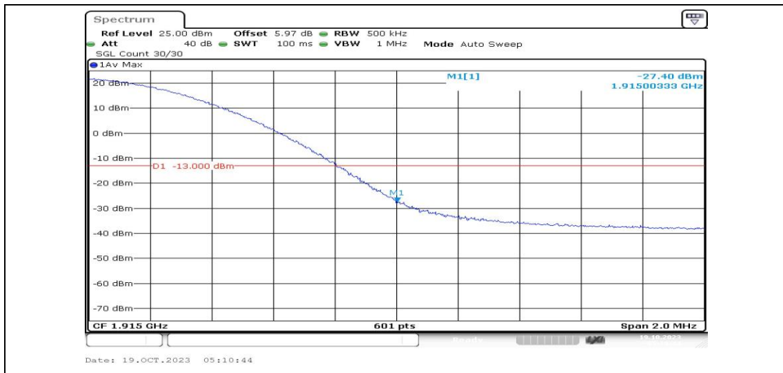
Band25-20MHz-QPSK-26590-1RB#99-PASS
