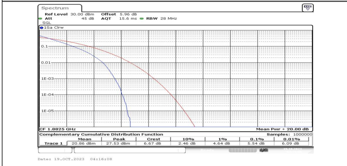
Band25-10MHz-QPSK-26365-50RB#0-PASS
