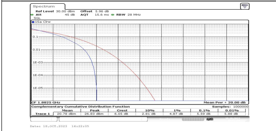
Band25-1.4MHz-QPSK-26365-6RB#0-PASS
