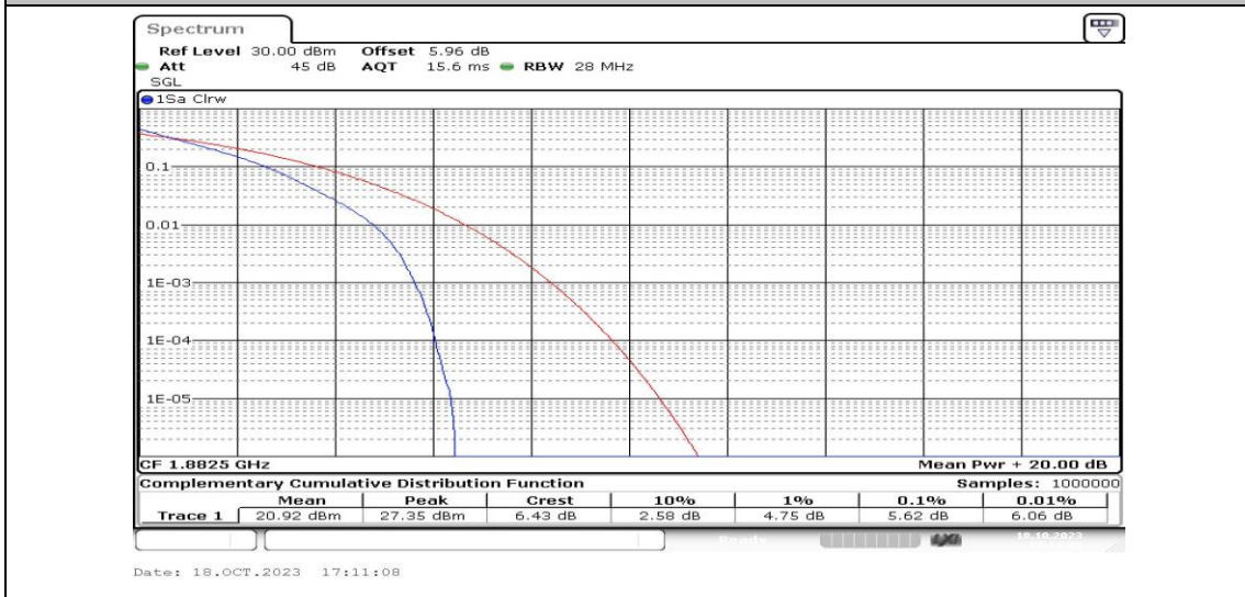
Band25-5MHz-QPSK-26365-25RB#0-PASS
