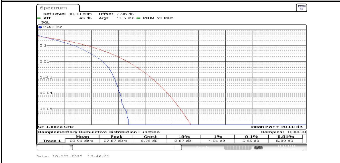
Band25-3MHz-QPSK-26365-15RB#0-PASS
