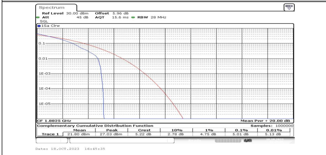
Band25-3MHz-QPSK-26365-1RB#0-PASS
