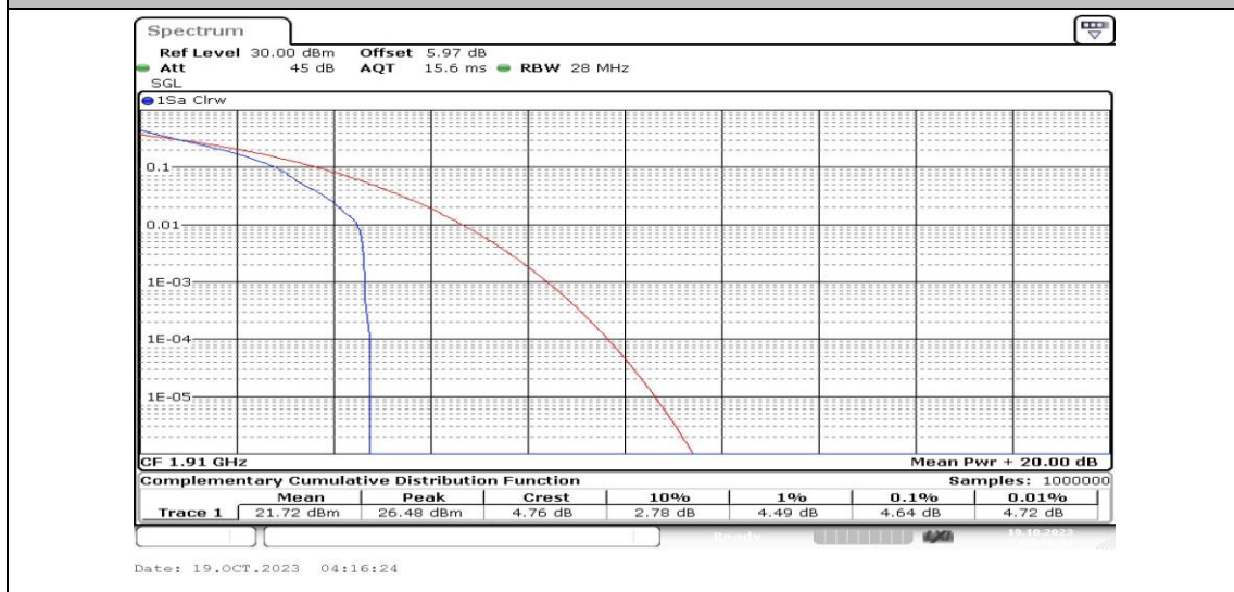
Band25-10MHz-QPSK-26640-1RB#0-PASS
