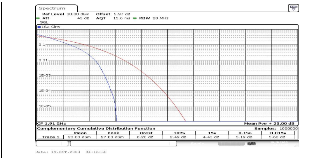
Band25-10MHz-QPSK-26640-50RB#0-PASS
