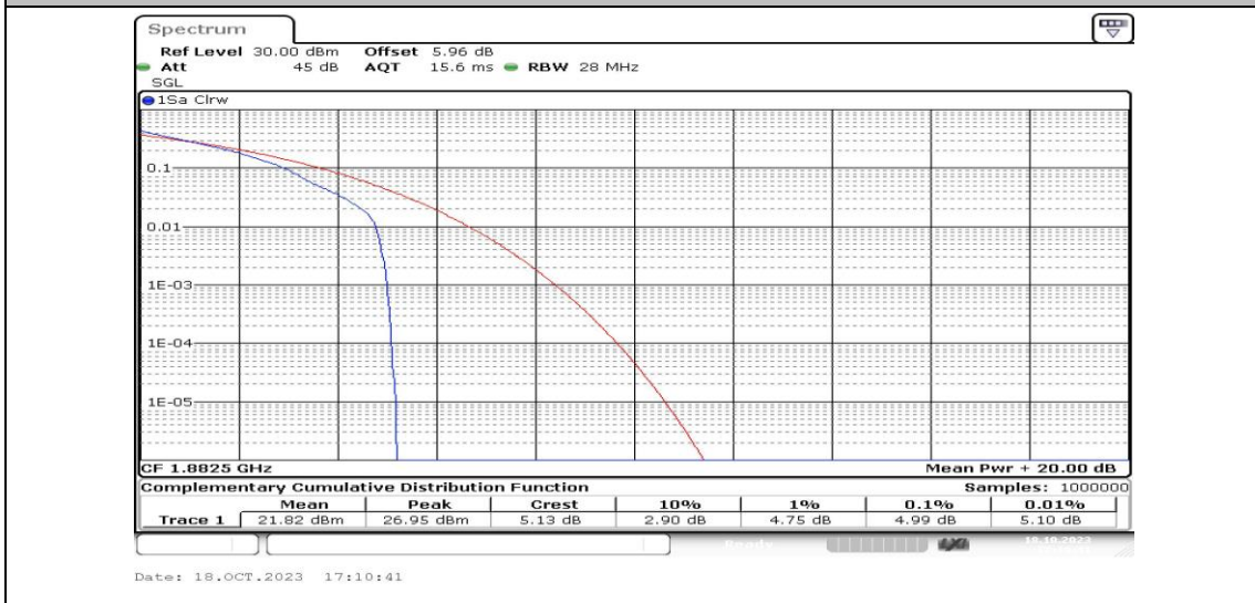
Band25-5MHz-QPSK-26365-1RB#0-PASS
