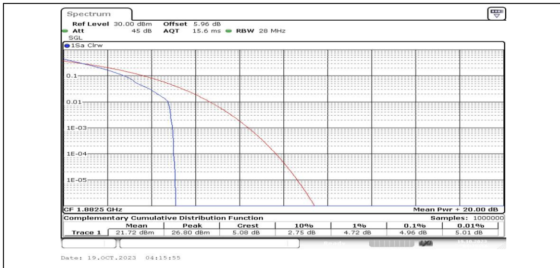
Band25-10MHz-QPSK-26365-1RB#0-PASS
