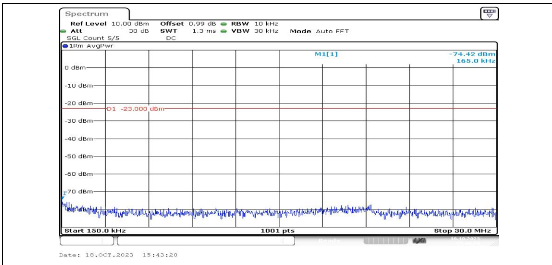
Band13-5MHz-QPSK-23230-1RB#0-Range2:0.15~30MHz-PASS
