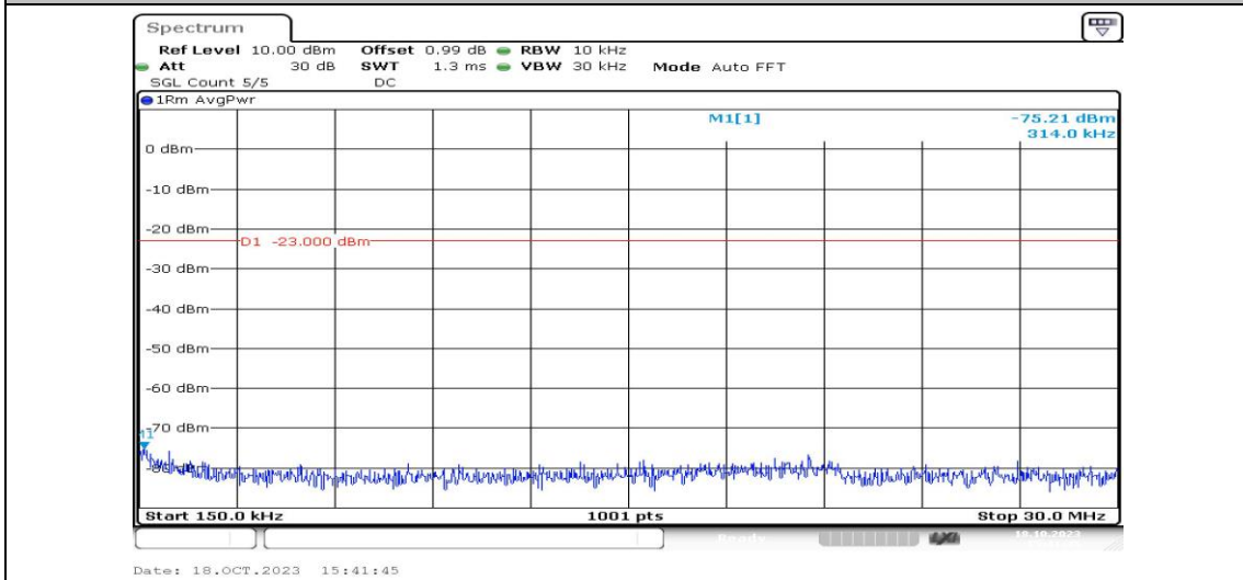
Band13-5MHz-QPSK-23205-1RB#0-Range2:0.15~30MHz-PASS
