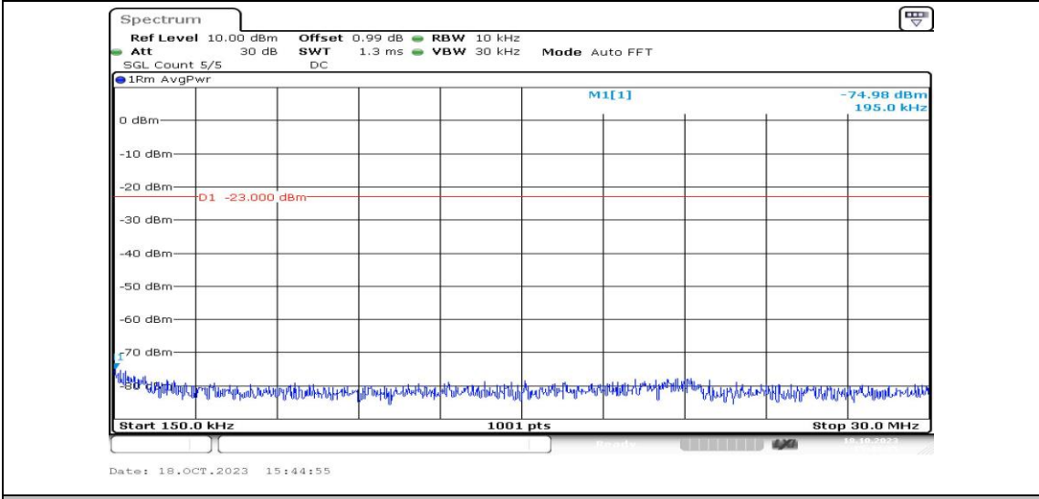
Band13-5MHz-QPSK-23255-1RB#0-Range2:0.15~30MHz-PASS
