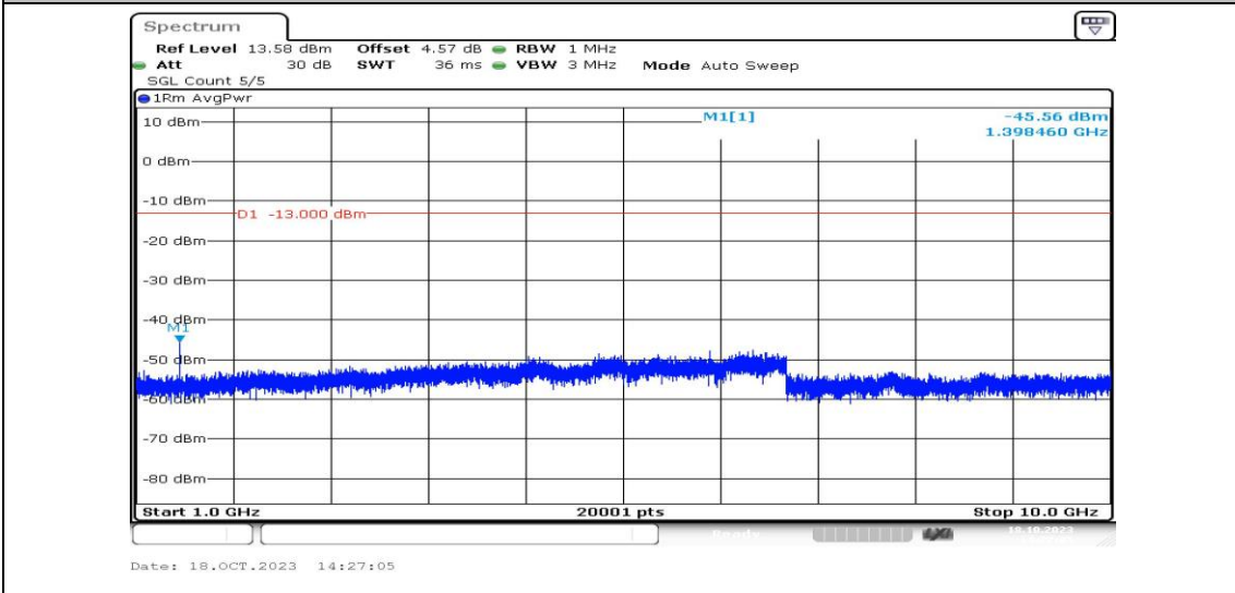
Band12-1.4MHz-QPSK-23017-1RB#0-Range4:1000~10000MHz-PASS
