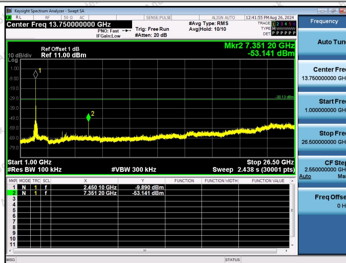
2.4G-Ant1-2451-1000~26500-PASS
