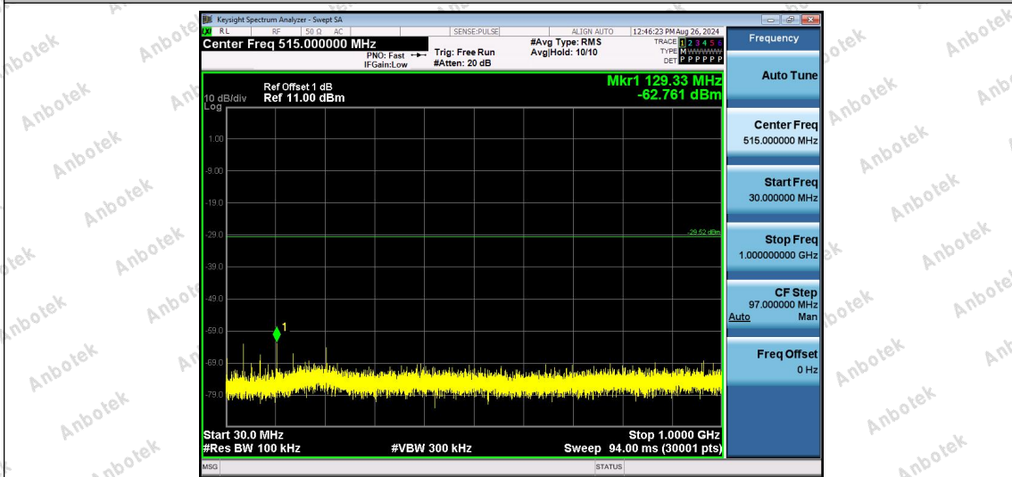
2.4G-Ant1-2475-30~1000-PASS
