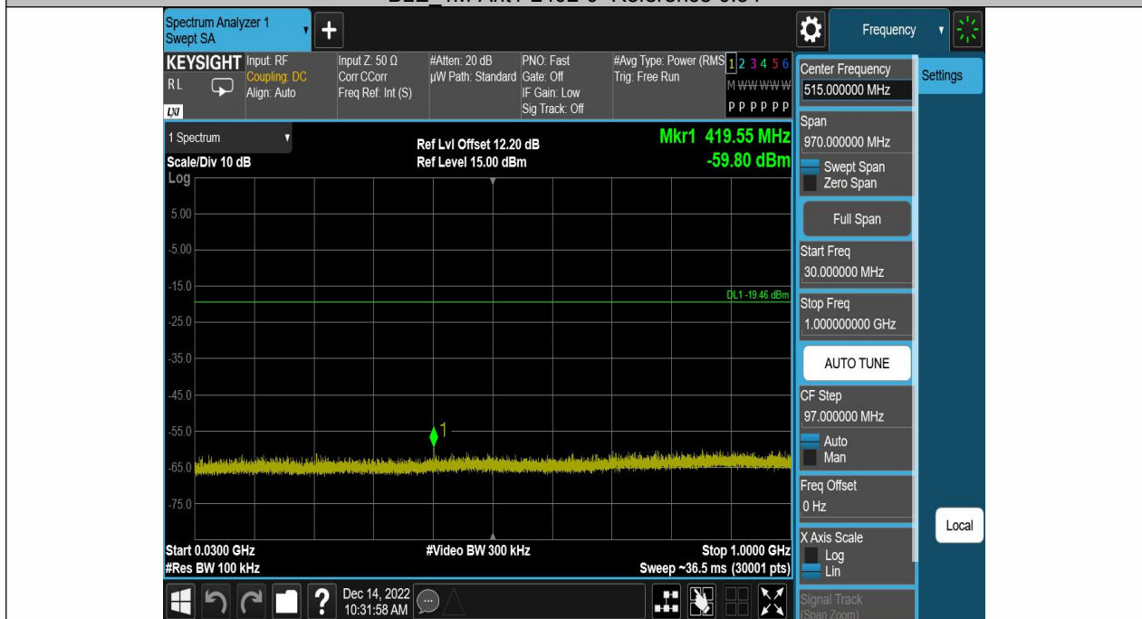
BLE_1M-Ant1-2402-30~1000-0.54
