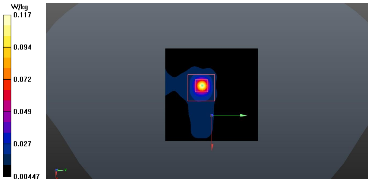
Fig. 2 LoRa Extremity
