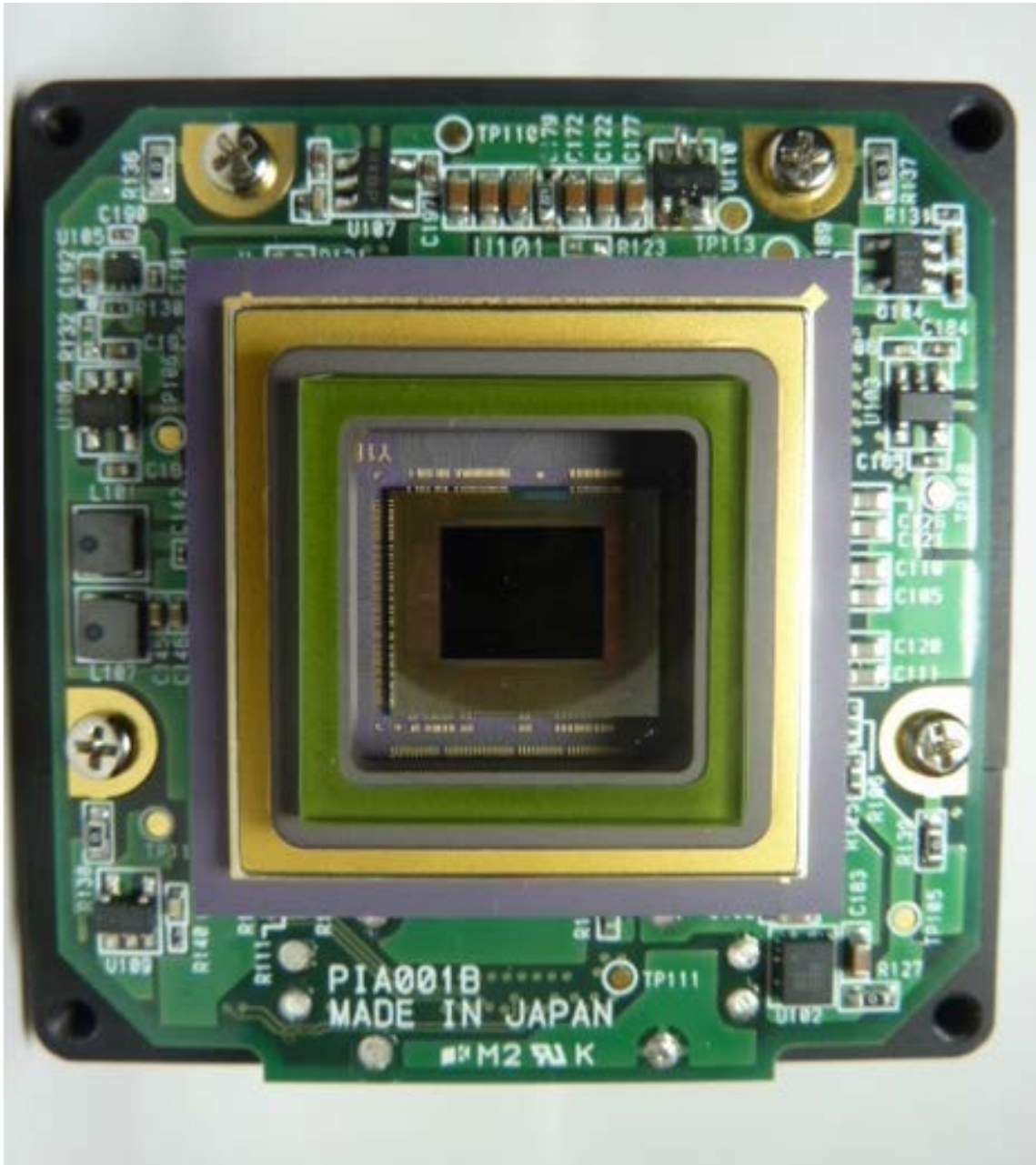
AssembledState_PCB1
