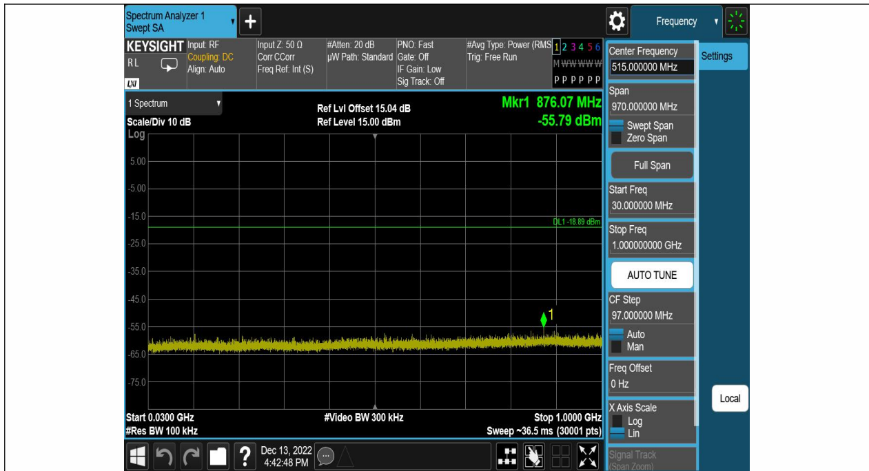
BLE_1M-Ant1-2440-30~1000-1.11
