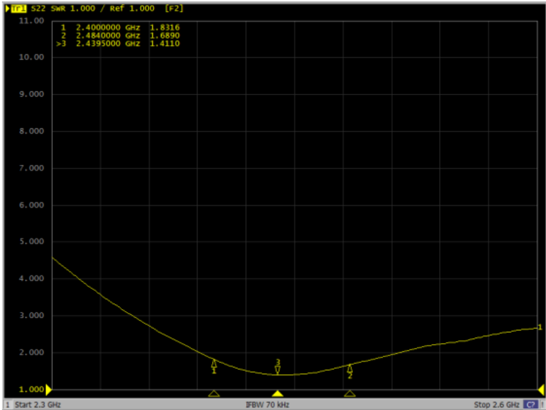
BT/WIFI VSWR
