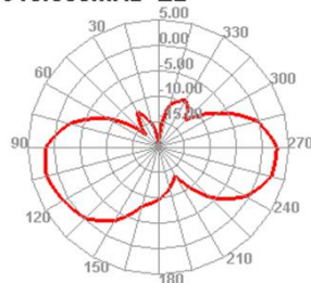
915.000MHz E2
