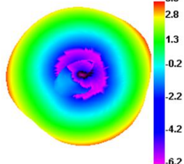
915.000MHz E1
