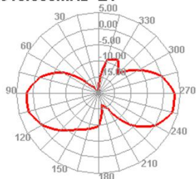
915.000MHz E1
