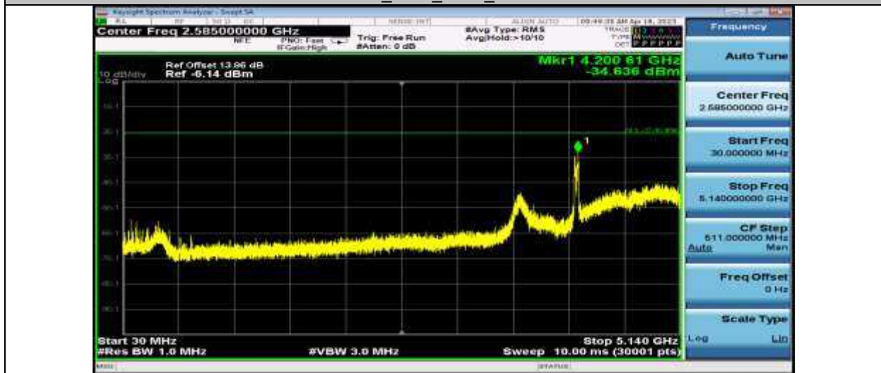
11N40SISO_Ant1_5230_30~5140
