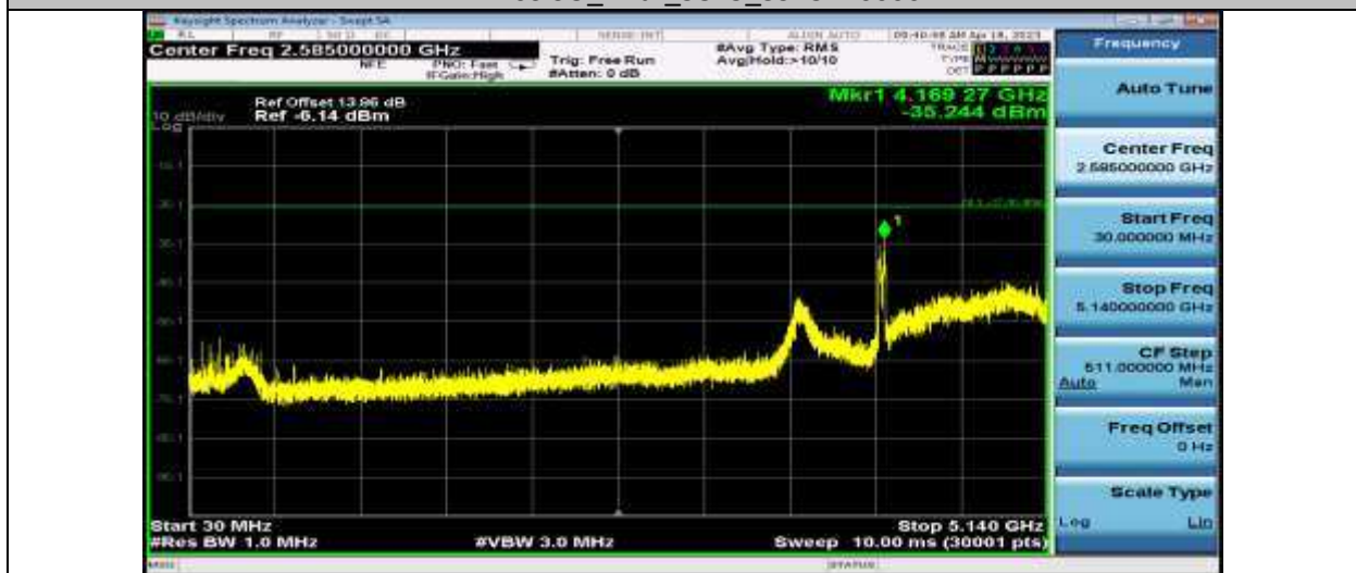
11N40SISO_Ant1_5190_30~5140
