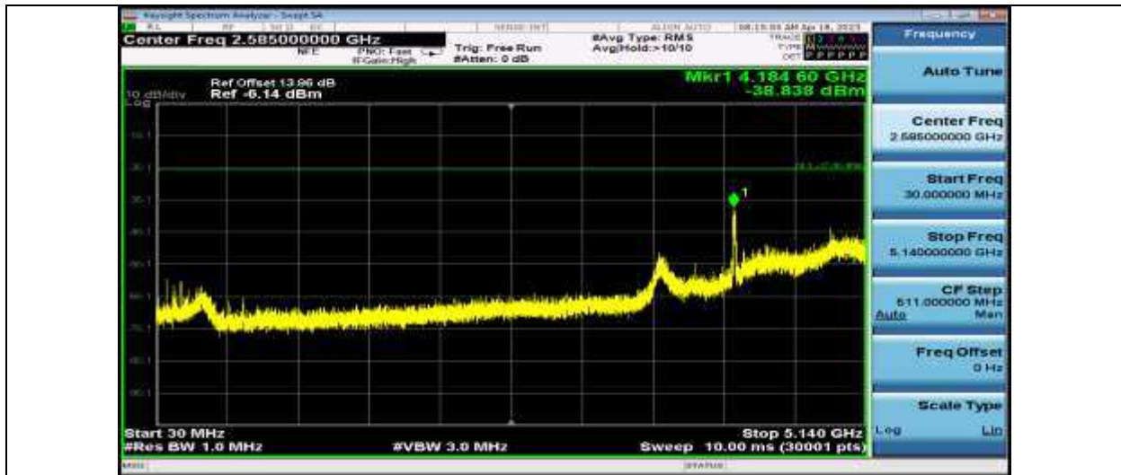
11A_Ant1_5240_30~5140
