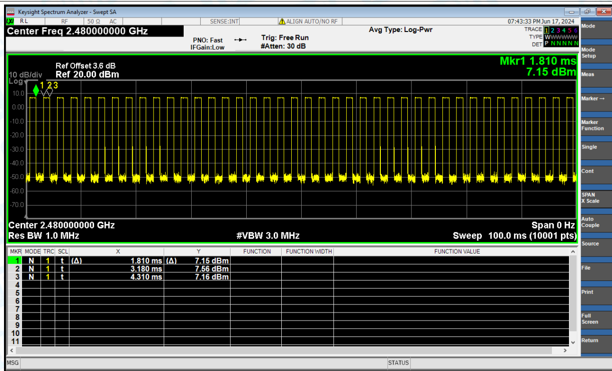
Duty Cycle NVNT BLE 2Mbps 2480MHz Ant1
