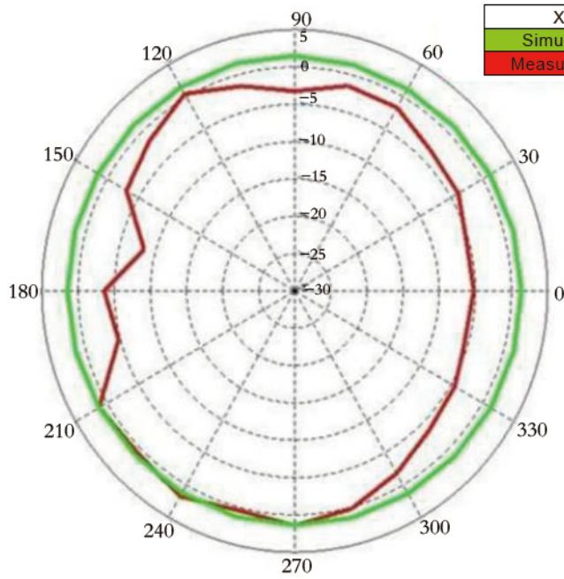
2480MHz
