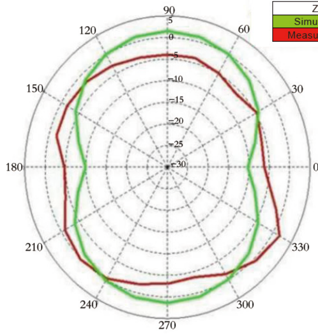
2480MHz
