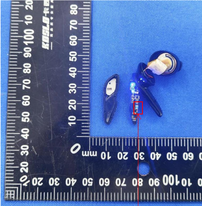
Antenna
