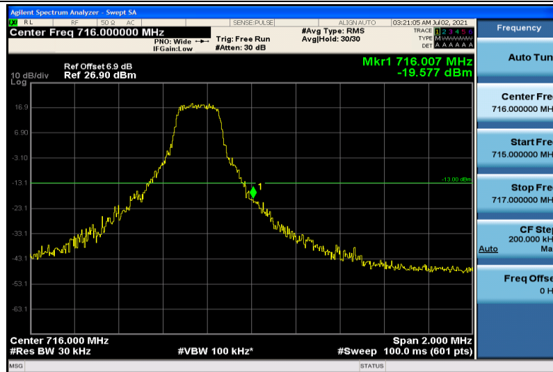
Band12-3MHz-QPSK-23165-1RB#14
