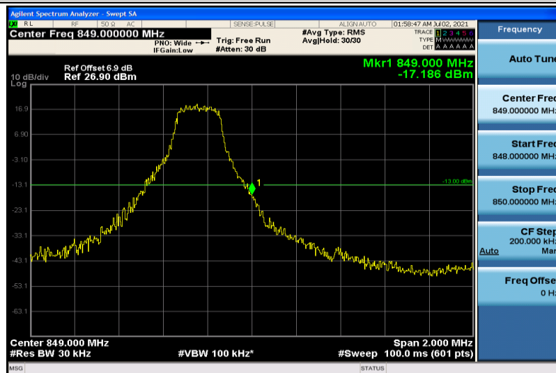
Band5-3MHz-QPSK-20635-1RB#14
