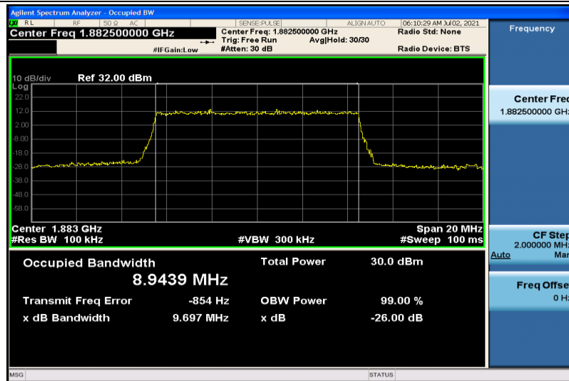
Band25-10MHz-QPSK-26365-50RB#0-8.9439
