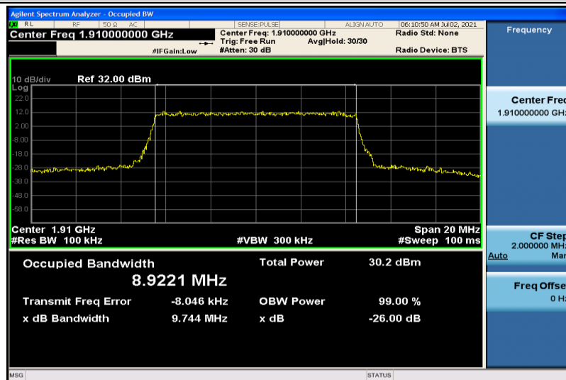
Band25-10MHz-QPSK-26640-50RB#0-8.9221
