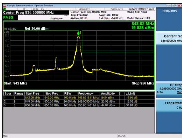
FDD26-Part 22-5MHz-QPSK-HCH-25RB#0
