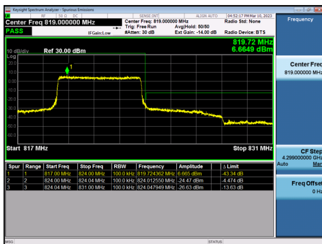
FDD26-Part 90-5MHz-QPSK-HCH-25RB#0
