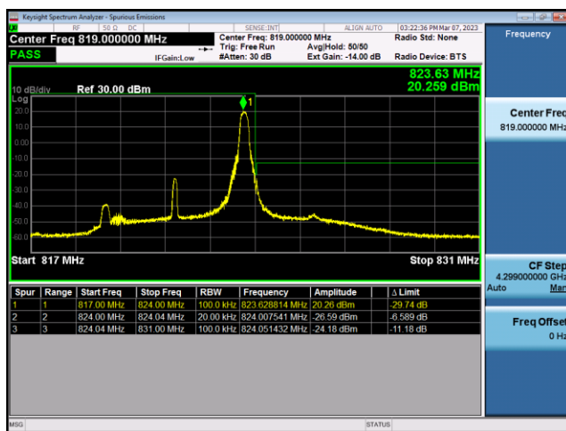
FDD26-Part 90-5MHz-QPSK-HCH-25RB#0
