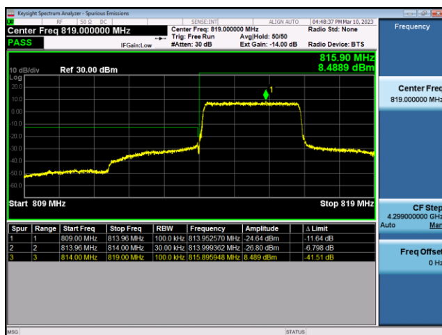
FDD26-Part 90-3MHz-QPSK-LCH-15RB#0
