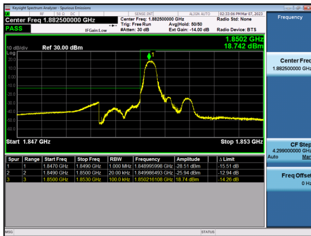
FDD25-1.4MHz-QPSK-LCH-6RB#0
