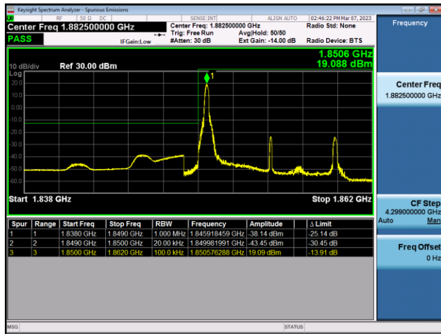
FDD25-10MHz-QPSK-LCH-50RB#0
