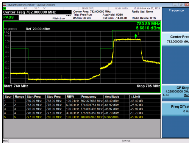
FDD13-10MHz-QPSK-MCH-1RB#0
