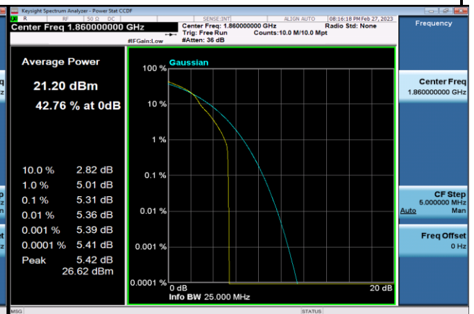
FDD25_LowRange_20MHz_1860_OneRB_high_Q16
