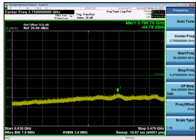
U-NII-2c ,Plot 2,30MHz~5470MHz-802.11 a(20MHz),5700MHz,Ant1
