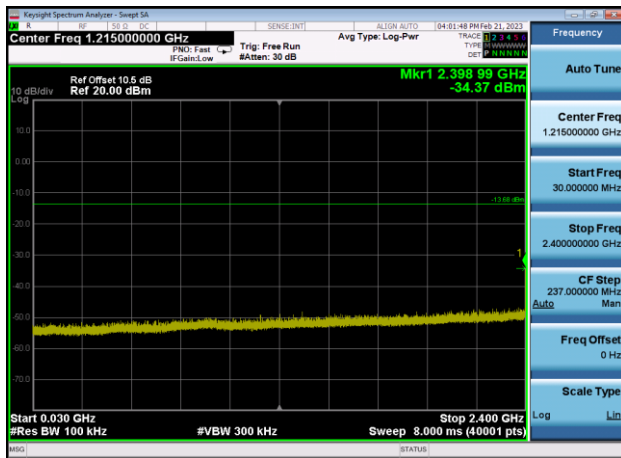
,Plot 3,30MHz~2400MHz-802.11b,2462MHz
