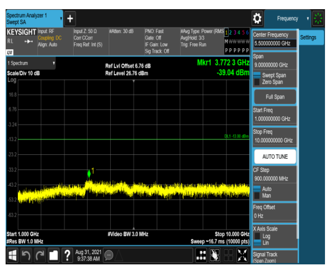
Band26-1.4MHz-QPSK-26797-1RB#0-Range2:1000~10000MHz
