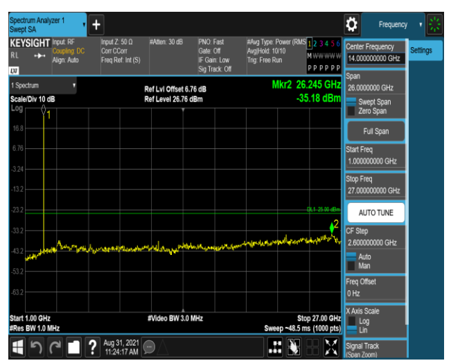
Band41-5MHz-QPSK-40640-1RB#0-Range1:30~1000MHz Band41-5MHz-QPSK-40640-1RB#0-Range2:1000~27000MHz
