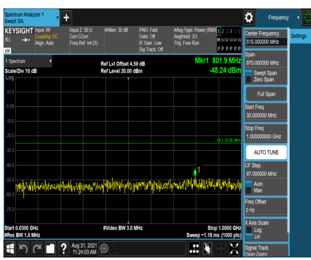
Band41-5MHz-QPSK-40640-1RB#0-Range1:30~1000MHz Band41-5MHz-QPSK-40640-1RB#0-Range2:1000~27000MHz
