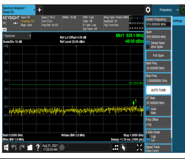
Band41-5MHz-QPSK-40640-1RB#0-Range1:30~1000MHz Band41-5MHz-QPSK-40640-1RB#0-Range2:1000~27000MHz
