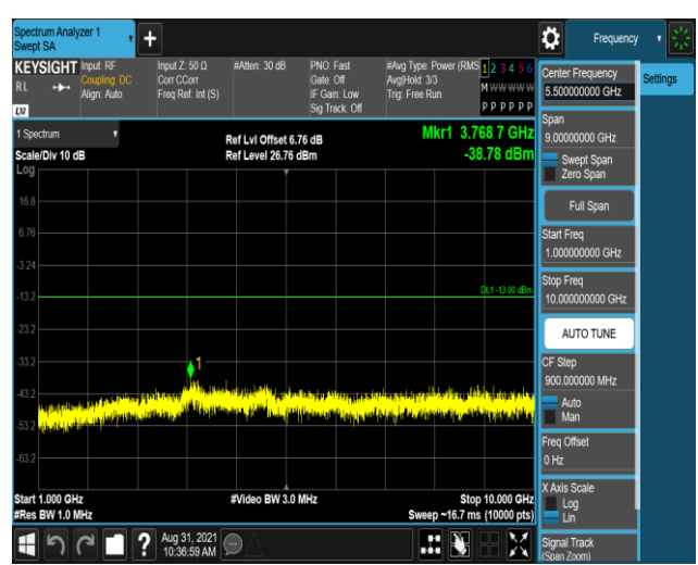
Band26-1.4MHz-QPSK-26797-1RB#0-Range2:1000~10000MHz
