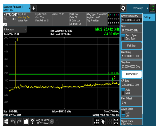
Band41-5MHz-QPSK-40640-1RB#0-Range1:30~1000MHz Band41-5MHz-QPSK-40640-1RB#0-Range2:1000~27000MHz
