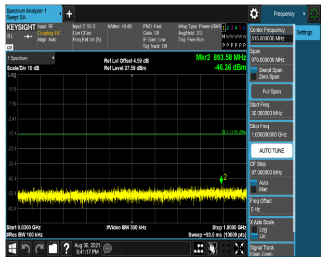
Band13-5MHz-QPSK-23230-1RB#0-Range1:30~1000MHz 00MHz
