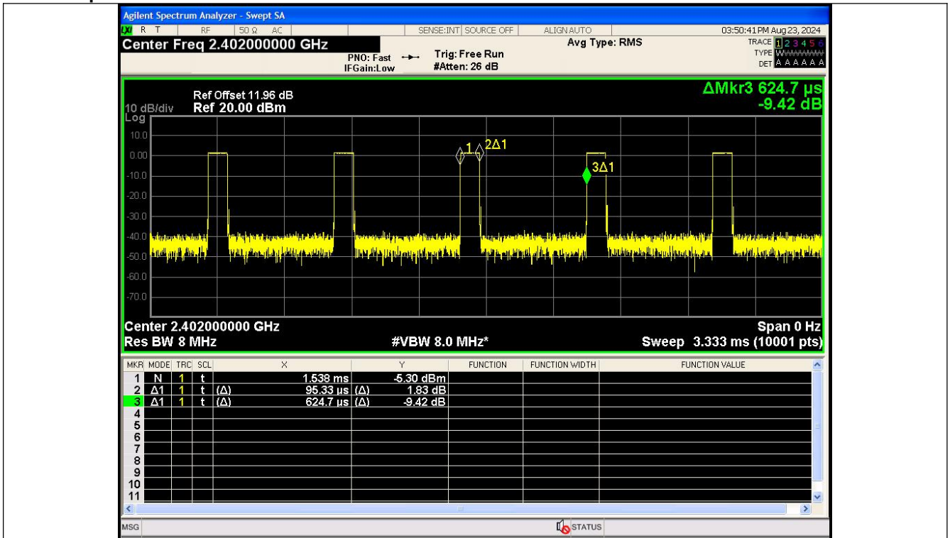
BLE 1M Channel 0
