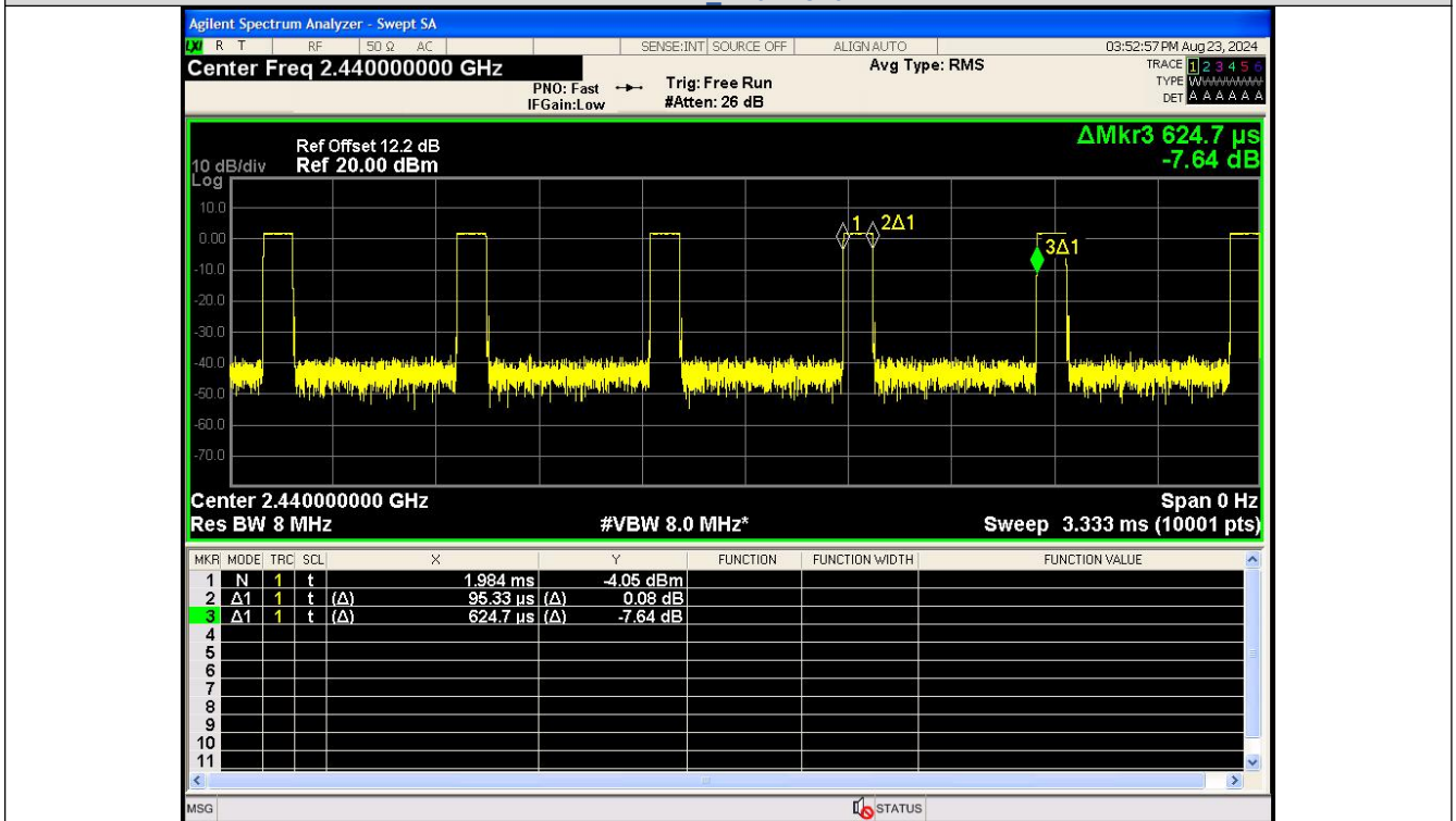
BLE 1M Channel 19
