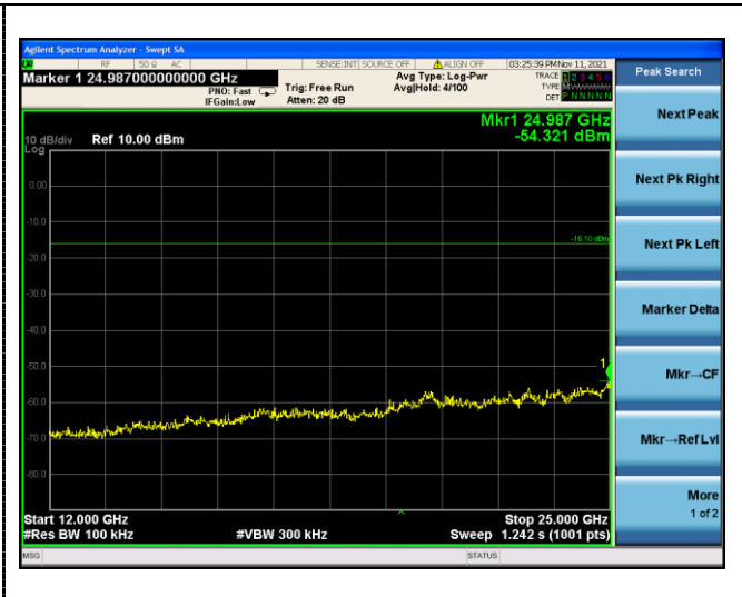
12GHz -25GHz
