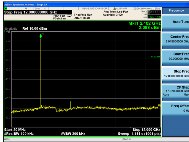
30MHz-12GHz
