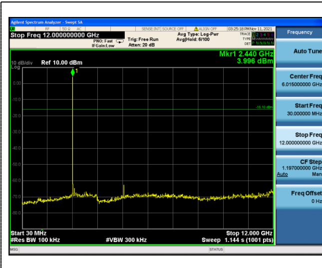
30MHz-12GHz
