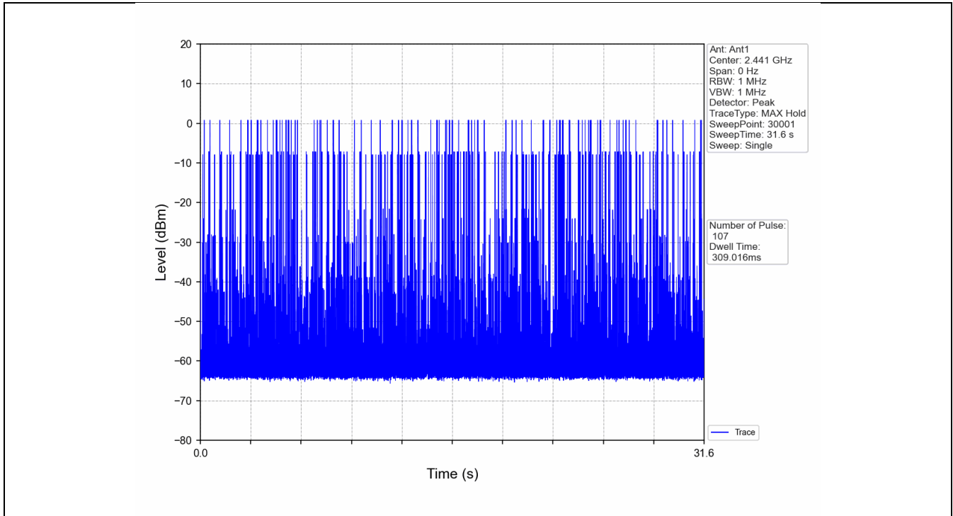
Pi/4DQPSK_2DH1_HOPP_Ant1_NTNV
