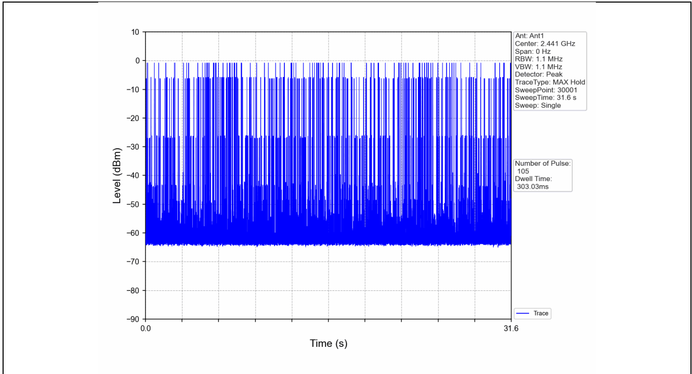
8DPSK_3DH1_HOPP_Ant1_NTNV
