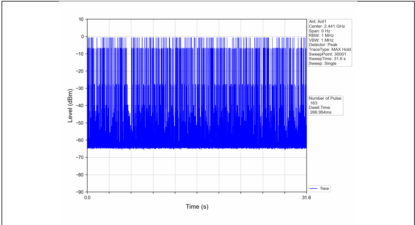
8DPSK_3DH5_HOPP_Ant1_NTNV
