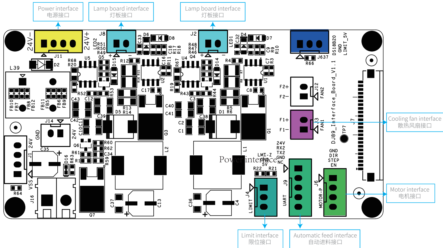
Adapter board circuit wiring diagram 转接板电路接线示意图
