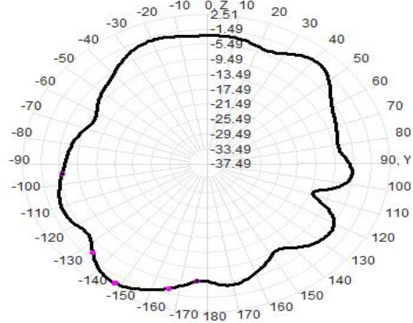
2420.0MHz Total(E2-YZ), Max= 0.08dBi
