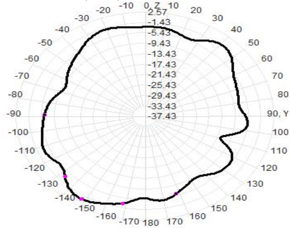
2430.0MHz Total(E2-YZ), Max= -0.21dBi
