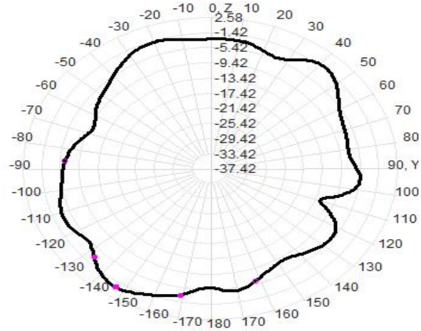
2435.0MHz Total(E2-YZ), Max= -0.37dBi
