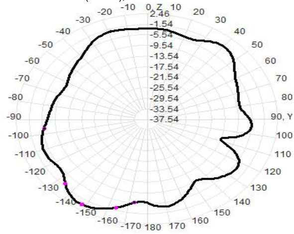
2410.0MHz Total(E2-YZ), Max= 0.26dBi
