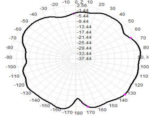
2445.0MHz Total(E1-XZ), Max= 2.56dBi
