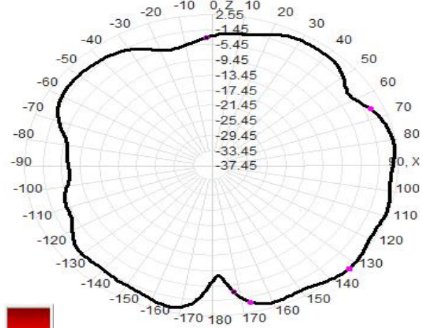
MHz Total(E1-XZ), Max= 2.55dBi
