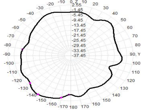
2455.0MHz Total(E2-YZ), Max= -0.56dBi
