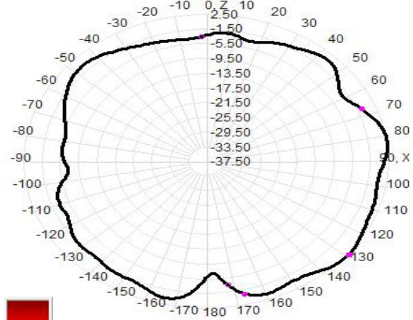
MHz Total(E1-XZ), Max= 2.50dBi
