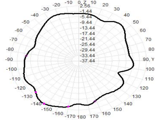
2440.0MHz Total(E2-YZ), Max= -0.50dBi
