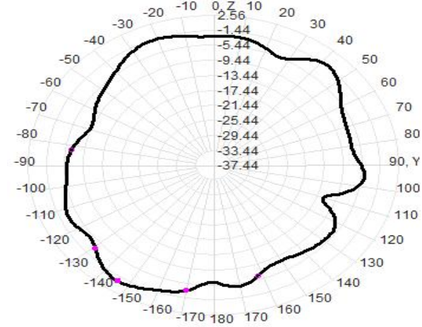
2445.0MHz Total(E2-YZ), Max= -0.55dBi
