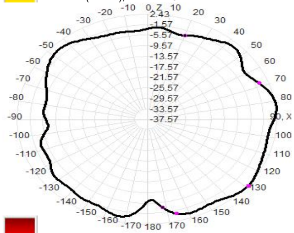
MHz Total(E1-XZ), Max= 2.43dBi
