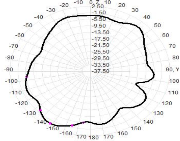
2415.0MHz Total(E2-YZ), Max= 0.20dBi
