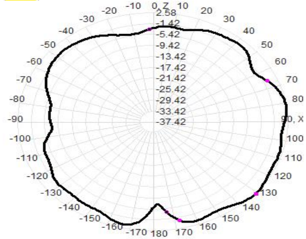
MHz Total(E1-XZ), Max= 2.58dBi
