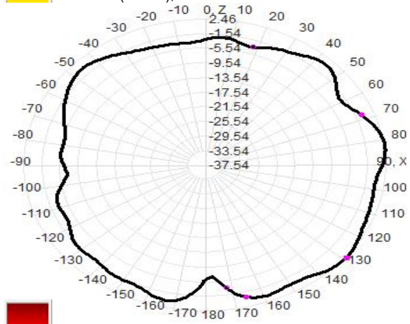
MHz Total(E1-XZ), Max= 2.46dBi
