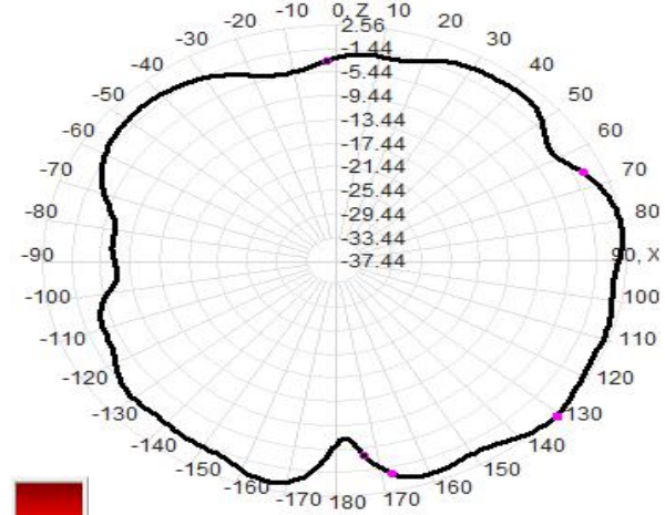
2440.0MHz Total(E1-XZ), Max= 2.56dBi
