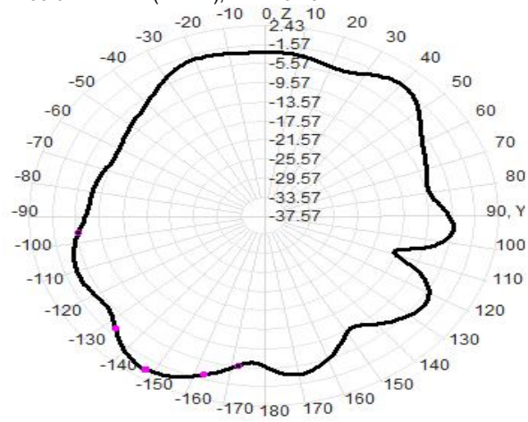
2405.0MHz Total(E2-YZ), Max= 0.28dBi
