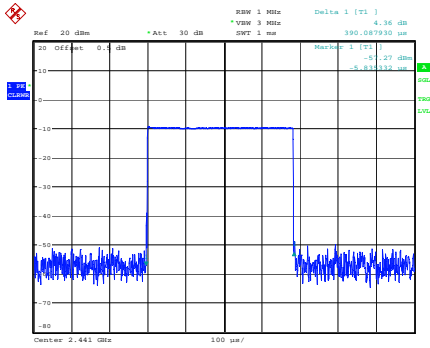
GFSK_Hopping_DH1 0.390ms
