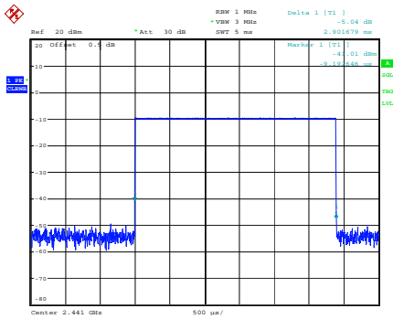
GFSK_Hopping_DH5 2.902ms
