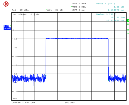
GFSK_Hopping_DH3 1.655ms
