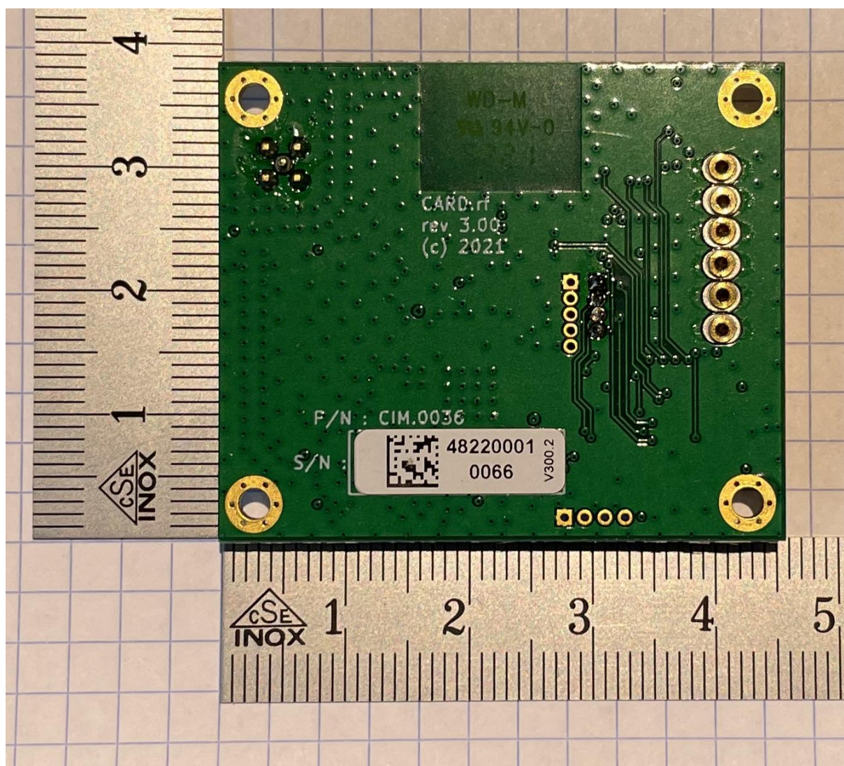
Module CRT.0036.915 bottom view:
