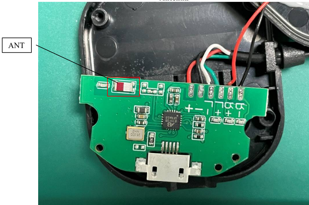
Antenna
