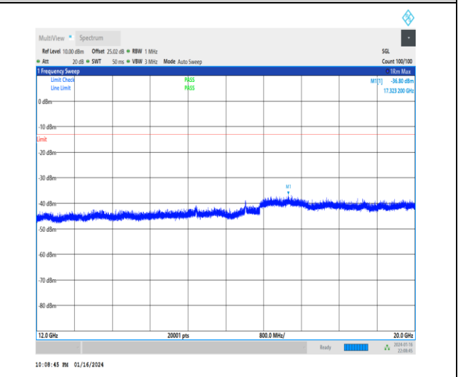
1-N26-824-849-15-20-M-1-DFT-PI2BPSK-Inner_1RB _Left-1@1-12000-20000-Ant0-17323.20--36.80--13-P ASS
