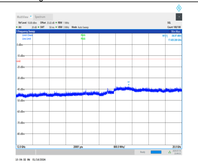
1-N26-824-849-15-20-L-1-DFT-PI2BPSK-Inner_1RB Left-1@1-12000-20000-Ant0-17402.40--36.97--13-PA SS
