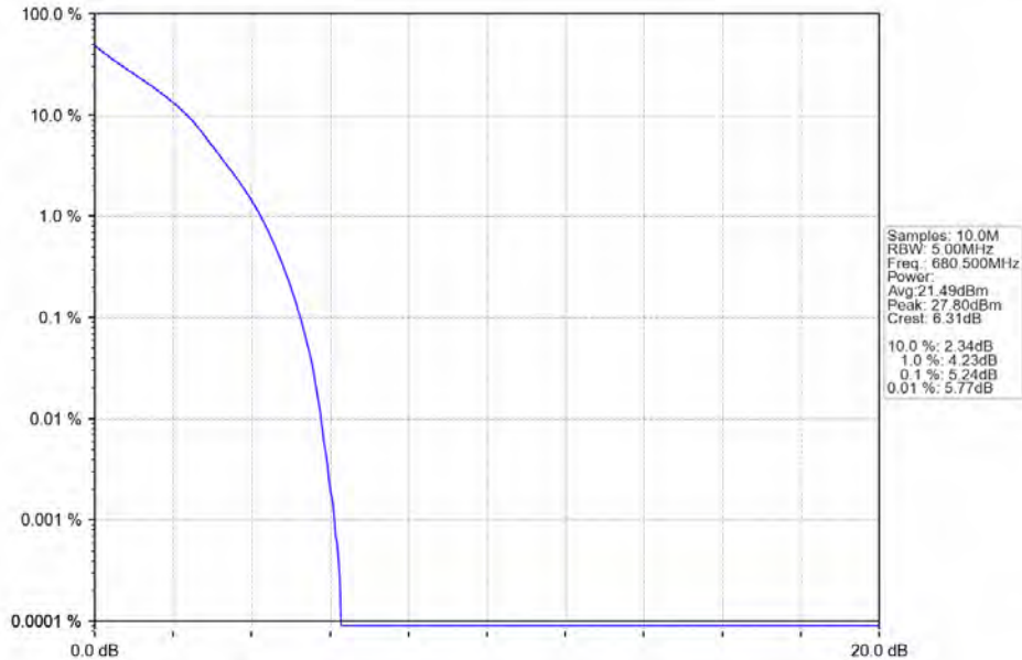
Band71 5MHz QPSK MCH 680.5MHz RB 25 0 NTV
