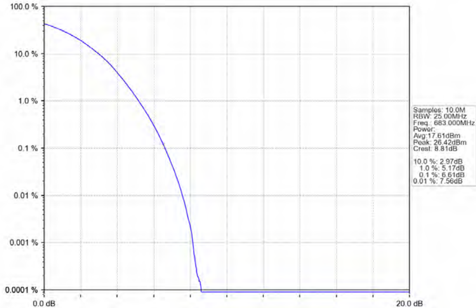
Band71 20MHz 256QAM MCH 683MHz RB 100 0 NTN
