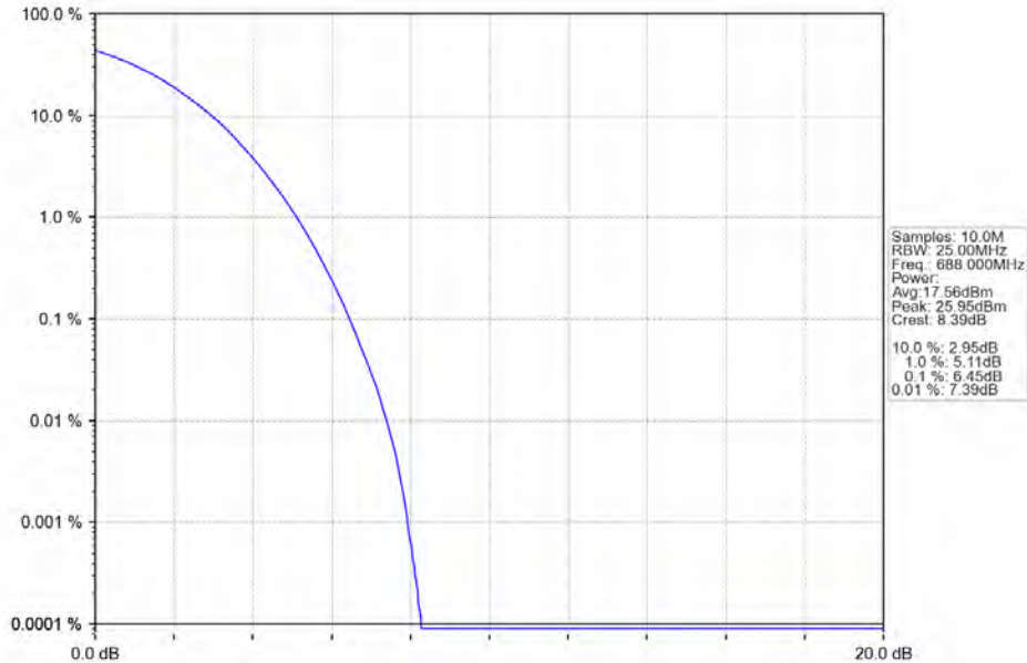
Band71 20MHz 256QAM HCH 688MHz RB 100 0 NTN
