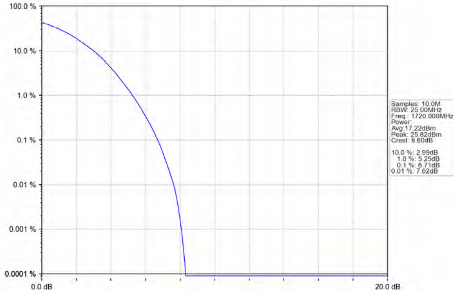
Band66 20MHz 256QAM LCH 1720MHz RB 100 0 NTN
