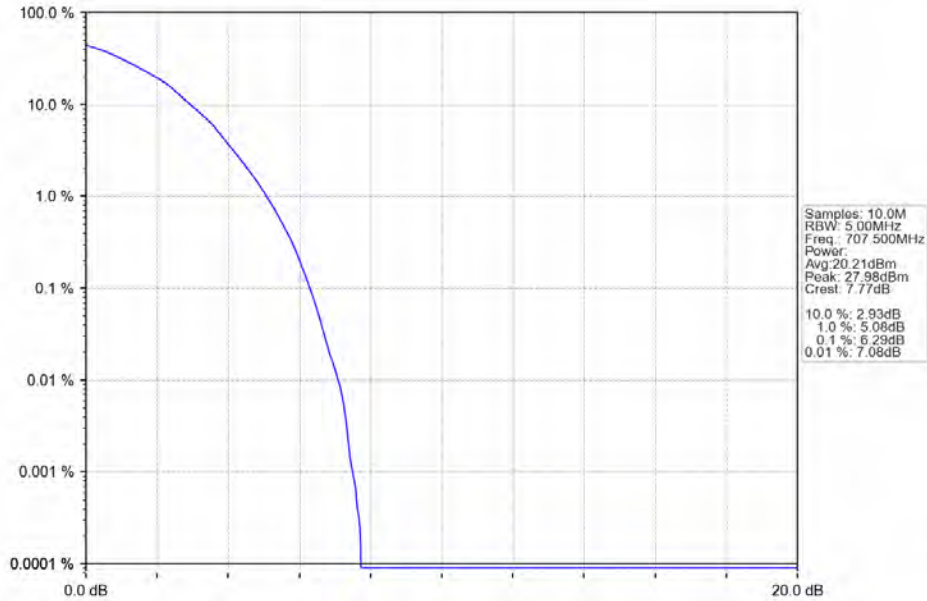
Band12 5MHz QPSK MCH 707.5MHz RB 25 0 NTV
