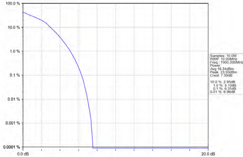
Band2 10MHz 16QAM HCH 1905MHz RB 50 0 NTV
