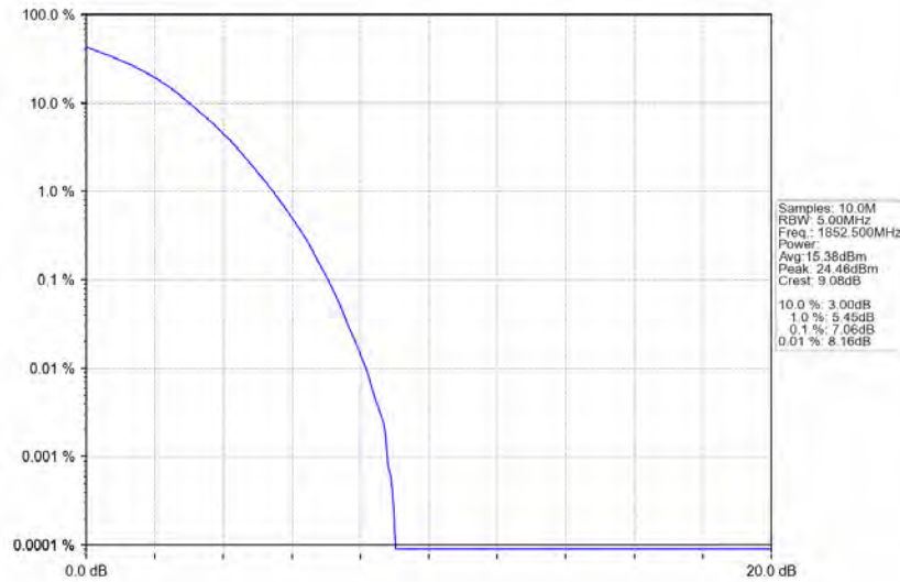
Band2 5MHz 256QAM LCH 1852.5MHz RB 25 0 NTV
