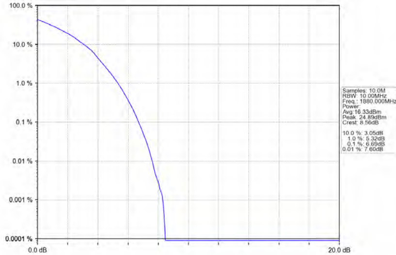
Band2 10MHz 64QAM MCH 1880MHz RB 50 0 NTV
