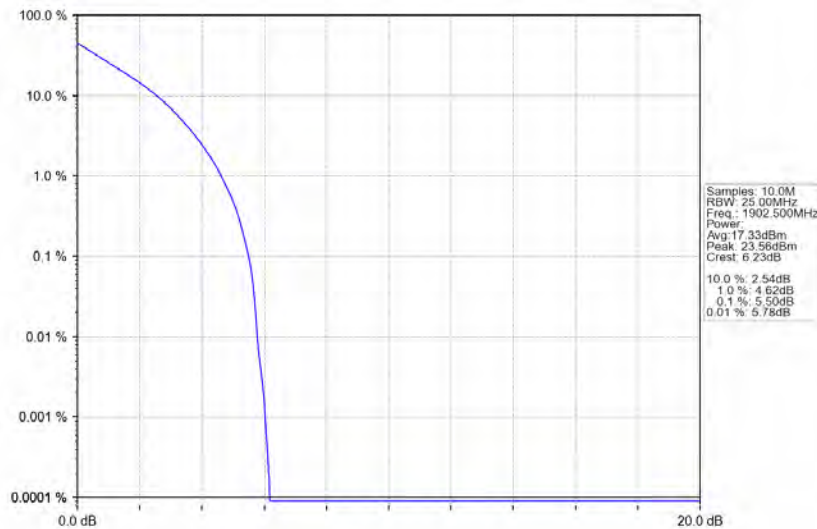
Band2 15MHz QPSK HCH 1902.5MHz RB 75 0 NTV
