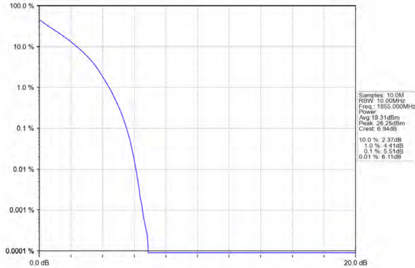
Band2 10MHz 16QAM LCH 1855MHz RB 50 0 NTV
