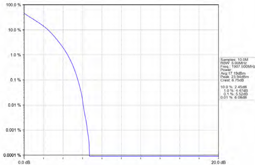
Band2 5MHz 64QAM HCH 1907.5MHz RB 25 0 NTV
