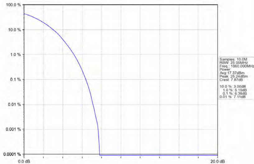
Band2 20MHz 64QAM LCH 1860MHz RB 100 0 NTN
