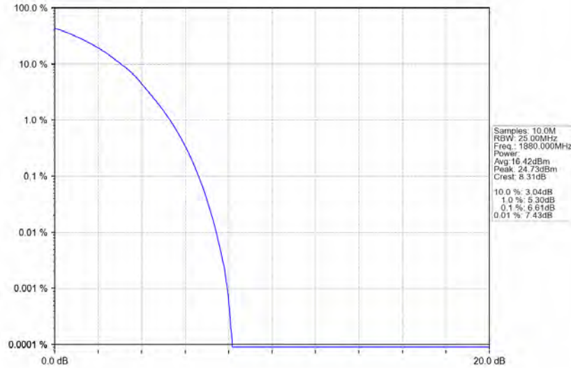
Band2 20MHz 64QAM MCH 1880MHz RB 100 0 NTN
