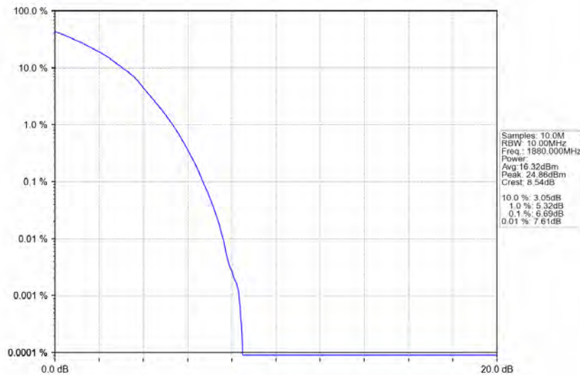
Band2 10MHz 16QAM MCH 1880MHz RB 50 0 NTV
