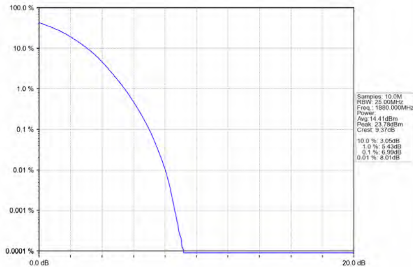
Band2 20MHz 256QAM MCH 1880MHz RB 100 0 NTNV
