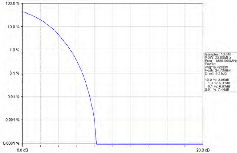
Band2 20MHz QPSK MCH 1880MHz RB 100 0 NTNV
