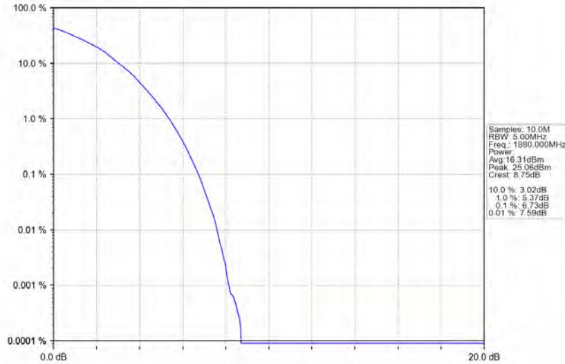
Band2 5MHz QPSK MCH 1880MHz RB 25 0 NTNV
