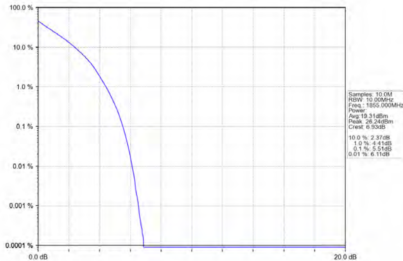
Band2 10MHz 64QAM LCH 1855MHz RB 50 0 NTV
