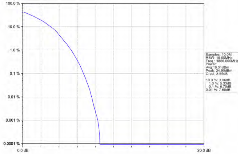
Band2 10MHz QPSK MCH 1880MHz RB 50 0 NTNV
