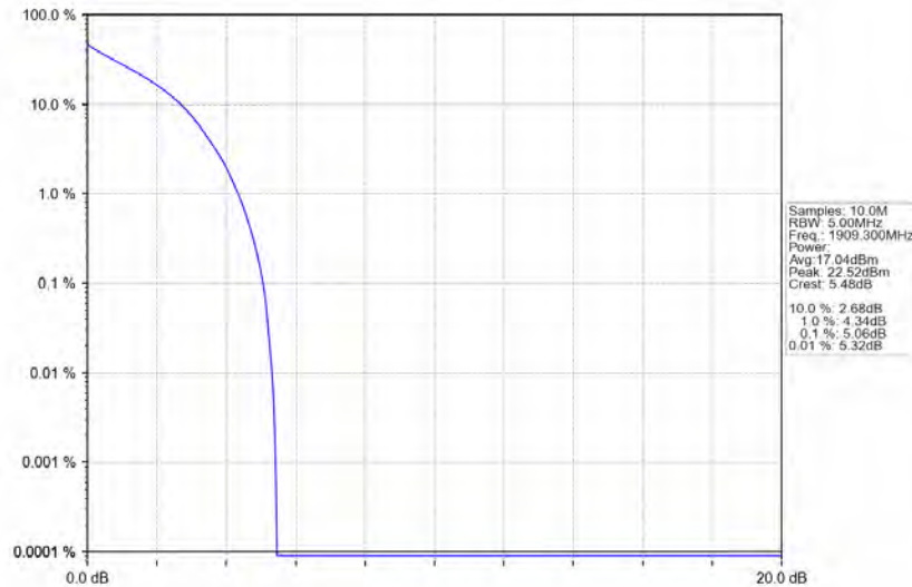
Band2 1.4MHz QPSK HCH 1909.3MHz RB 6 0 NTNV
