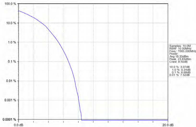
Band2 10MHz 64QAM HCH 1905MHz RB 50 0 NTV
