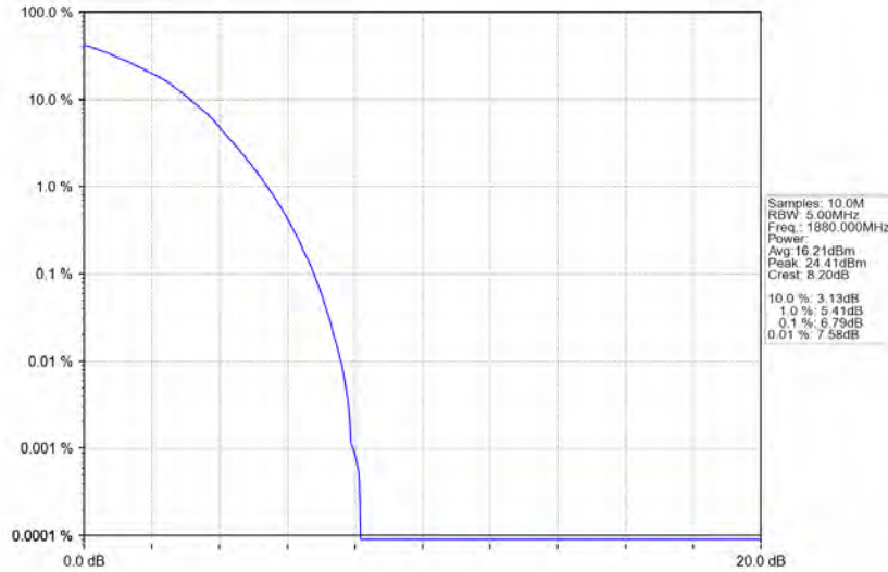
Band2 3MHz QPSK MCH 1880MHz RB 15 0 NTNV
