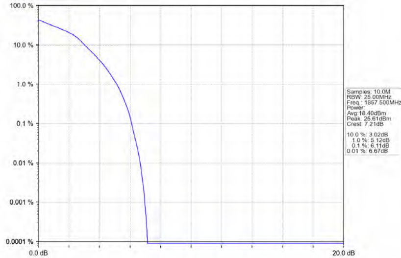
Band2 15MHz 16QAM LCH 1857.5MHz RB 75 0 NTV
