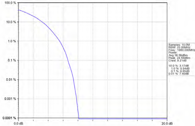
Band2 15MHz QPSK MCH 1880MHz RB 75 0 NTV
