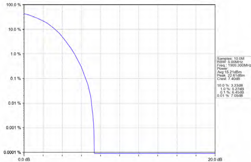
Band2 1.4MHz 64QAM HCH 1909.3MHz RB 6 0 NTV
