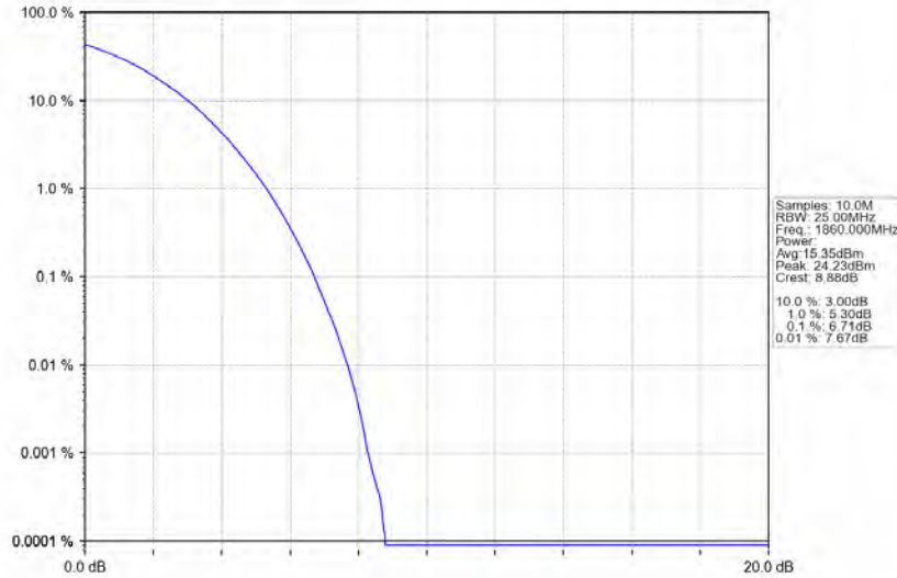
Band2 20MHz 256QAM LCH 1860MHz RB 100 0 NTNV
