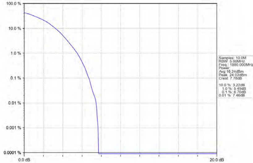
Band2 1.4MHz QPSK MCH 1880MHz RB 6 0 NTNV
