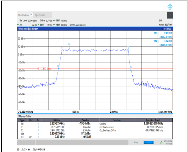
1-N77-3700-3980-30-10-M-9-CP-256QAM-Outer_Fu II-24@0-Ant4-8.58-9.320-≤10-PASS
