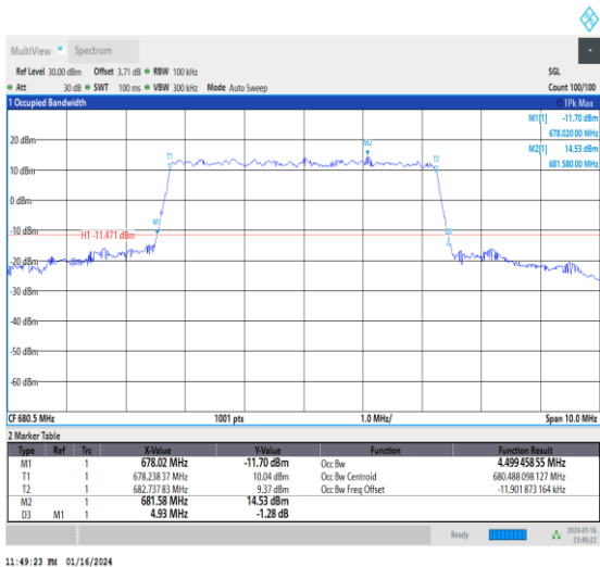
1-N71-15-5-M-7-CP-16QAM-Outer_Full-25@0-Ant0-4 4.499-4.930-≤5-PASS
