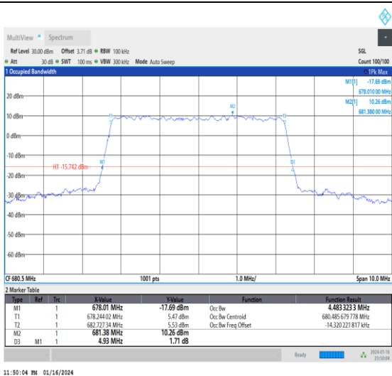
1-N71-15-5-M-9-CP-256QAM-Outer_Full-25@0-Ant0 -4.483-4.930-≤5-PASS
