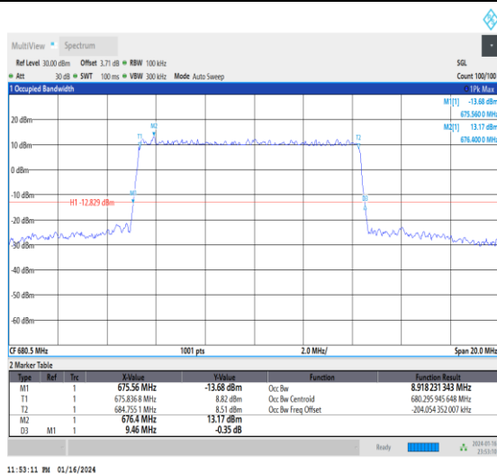
1-N71-15-10-M-3-DFT-16QAM-Outer_Full-50@0-Ant0 0-8.918-9.460-≤10-PASS
