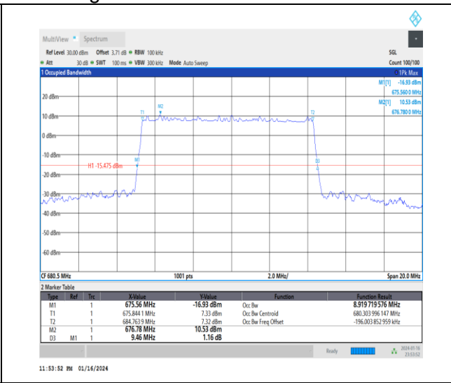
1-N71-15-10-M-5-DFT-256QAM-Outer_Full-50@0-A nt0-8.92-9.460-≤10-PASS
