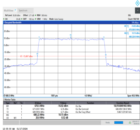
1-N71-15-20-M-9-CP-256QAM-Outer_Full-106@0-Ant0 nt0-18.919-20.000-≤20-PASS
