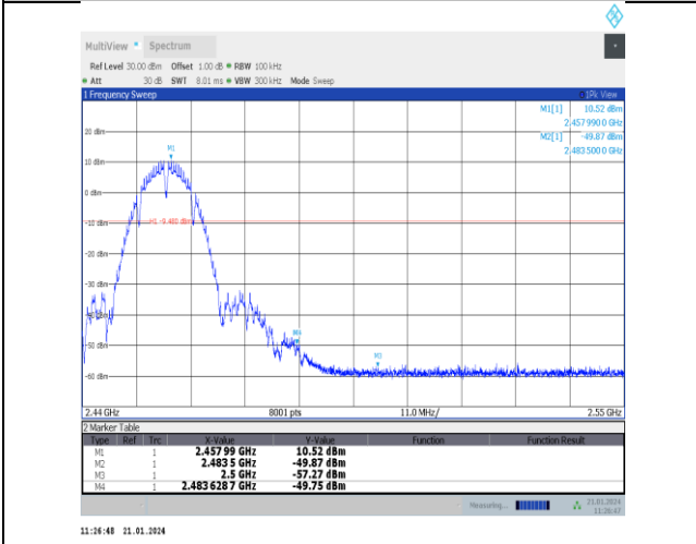
11b-Ant5-2457-PASS
