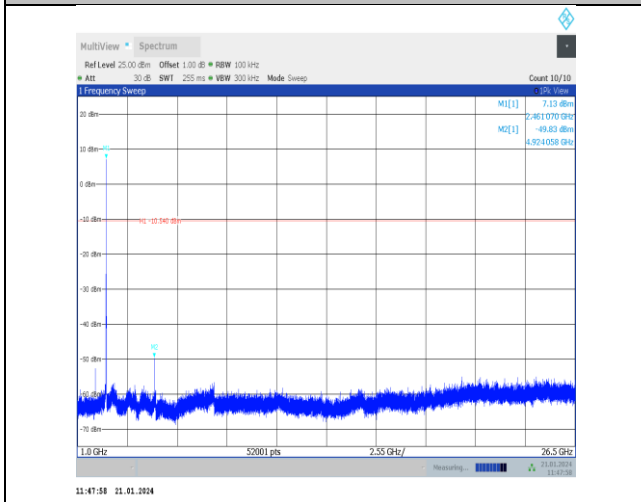
11b-Ant5-2462-1000~26500-PASS
