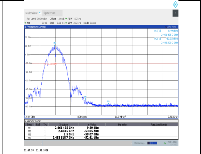
11b-Ant5-2462-PASS
