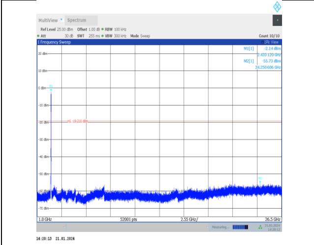
11n40ISO-Ant5-2442-1000~26500-PASS
