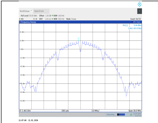
11b-Ant5-2462-0~Reference-PASS
