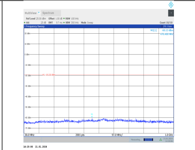
11n40ISO-Ant5-2442-30~1000-PASS
