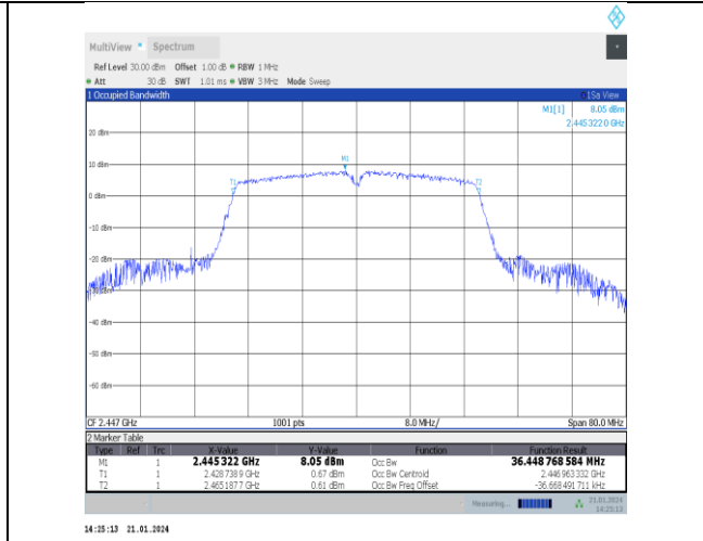
11n40ISO-Ant5-2447
