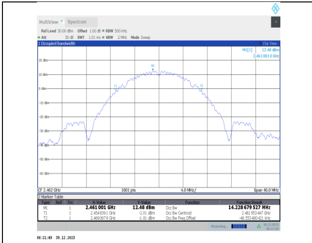
11b-Ant5-2462
