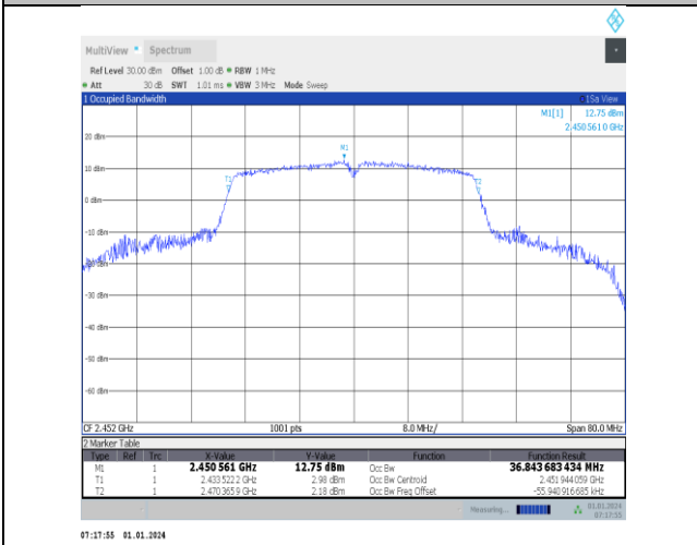
11n40ISO-Ant5-2452
