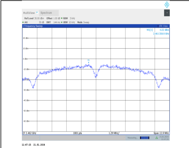
11b-Ant5-2462-PASS
