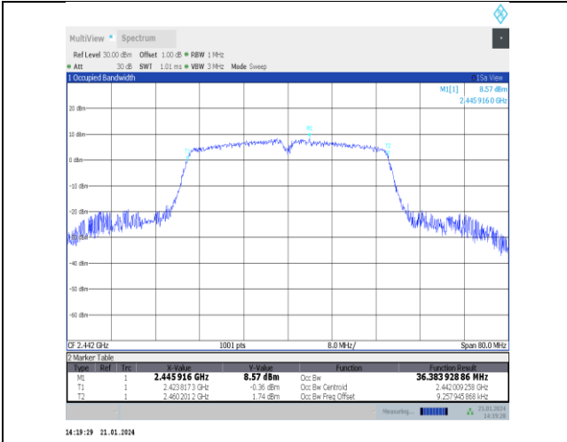
11n40ISO-Ant5-2442
