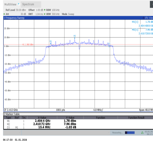
11n20ISO-Ant5-2412-PASS
