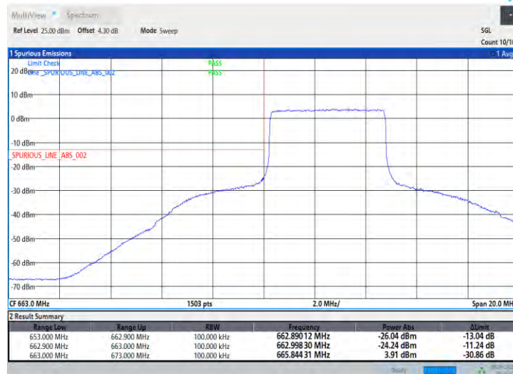
Band71-5MHz-QPSK-133147-25RB#0
