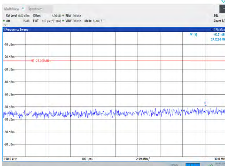
Band71-20MHz-QPSK-133222-1RB#0-Range2:0.15~30MHz
